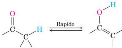
Tautomero chetonico
