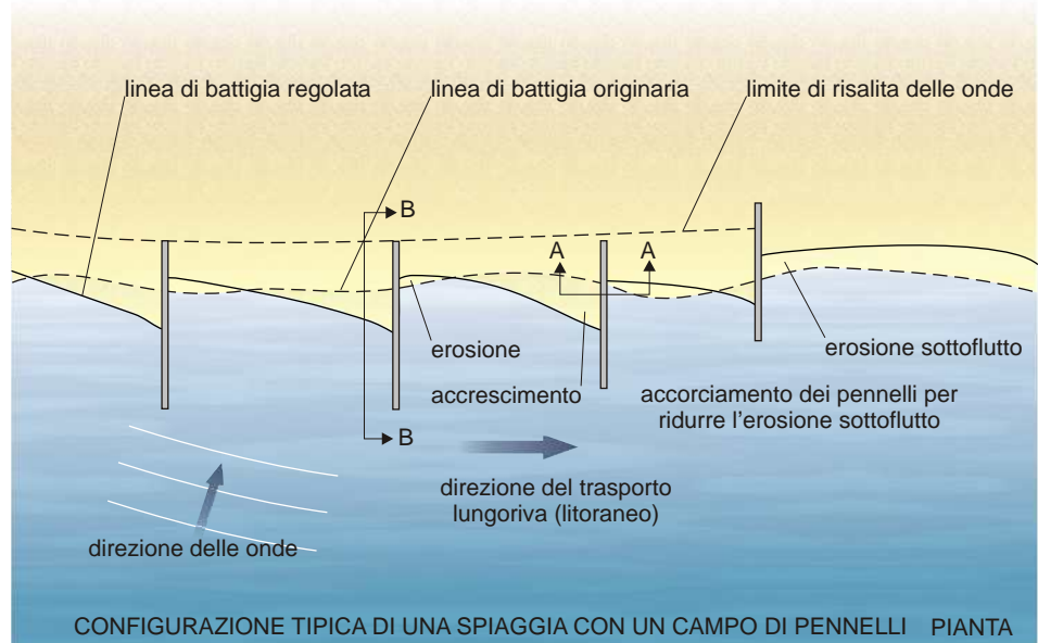
Figura 4.2.2: Esempio di "campo di pennelli". Un sistema di pennelli può favorire la formazione di una spiaggia solamente se le onde e le correnti trasportano una sufficiente quantità di sedimenti. Per ridurre l'erosione sottoflutto, gli elementi terminali di ogni campo di pennelli devono essere progressivamente accorciati.
