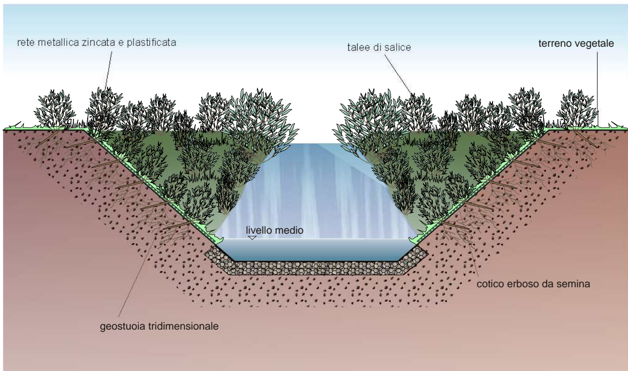
Figura 5.2.2: Rivestimento in rete metallica a doppia torsione e geostuoia tridimensionale.
