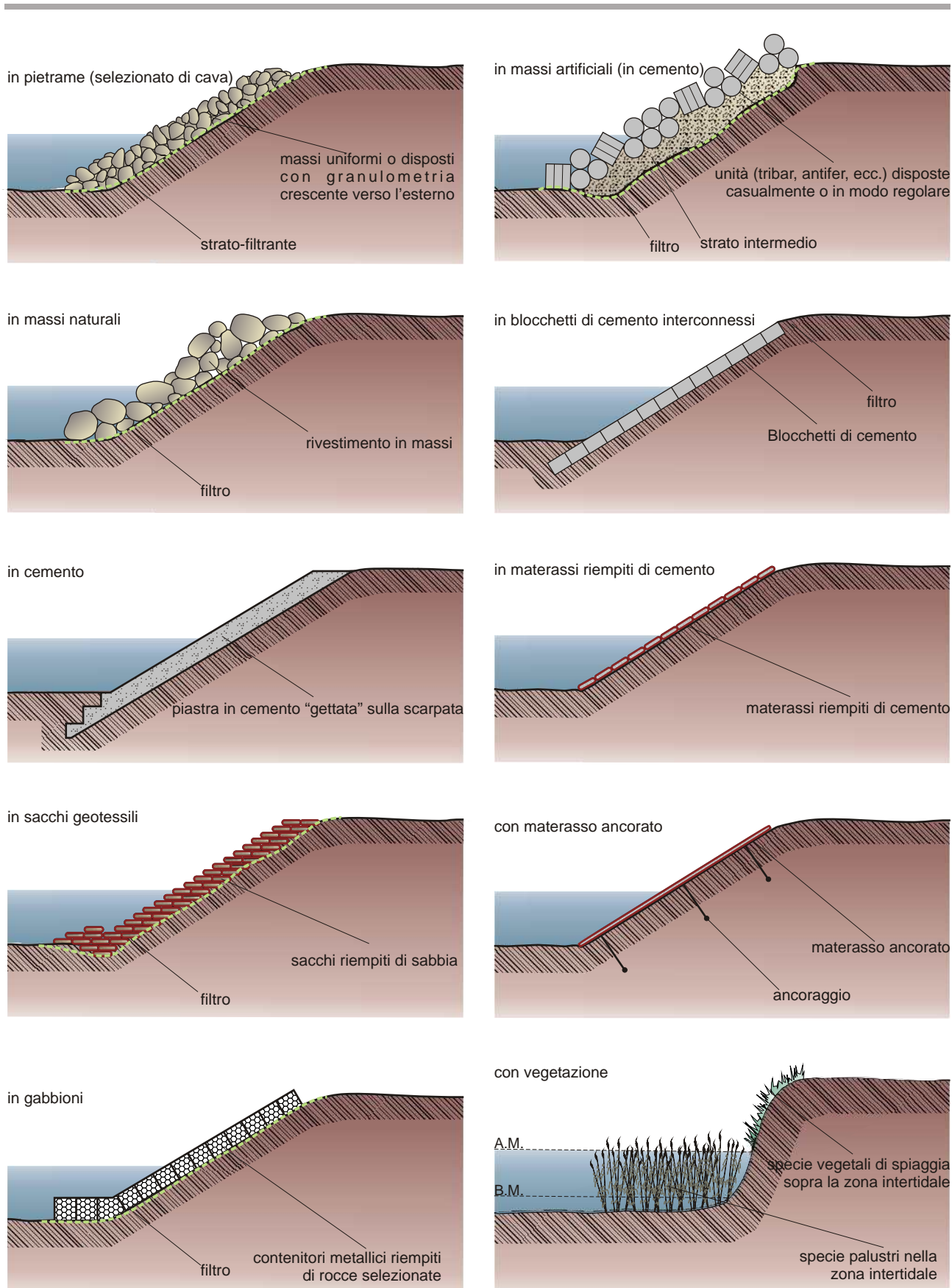
Figura 4.3.6: Tipi di rivestimento. L'estremità inferiore del rivestimento dovrebbe sempre essere sepolta al di sotto del fondale per evitare problemi di scalzamento alla base; inoltre è opportuno disporre un filtro tra i massi di protezione e il terreno della scarpata, per prevenire cedimenti differenziali e distribuire meglio il peso delle singole unità.
