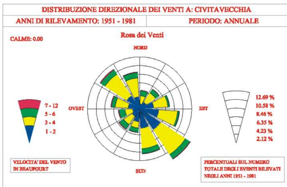
Figura 2.2.2: Il regime dei venti in una data località costiera può essere definito mediante distribuzioni di frequenza per settori direzionali e campi di velocità, con riferimento a periodi di osservazione possibilmente pluriennali. Come dati di base per la definizione del regime del vento vanno assunti quelli forniti da stazioni anemometriche presenti nella zona in esame.
