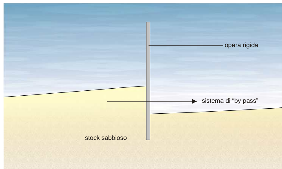
Figura 4.4.7: Schema di applicazione di un sistema di by pass per il refluito di sabbie litoranee accumulate a ridosso di un'opera antropica.
