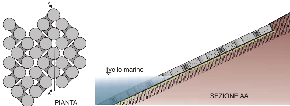
Figura 4.3.23: Rivestimento tipo Elbloc.
