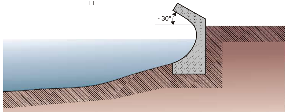
Figura 4.3.33: Esempio di muro concavo con parapetto inclinato di 30°. La sua funzione principale è quella di evitare che le onde in risalita scavalchino il coronamento e producano erosione a tergo, evitando anche l'ingresso di acqua su strade o vicino ad edifici.
