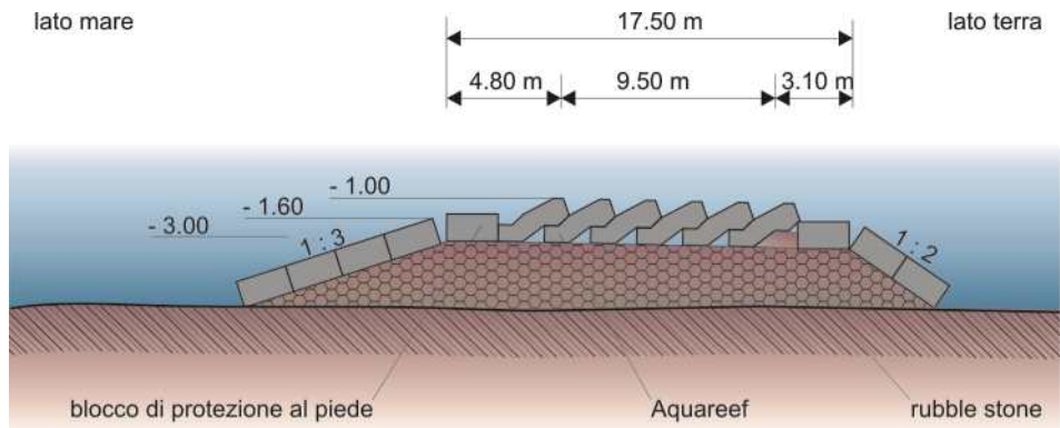
Figura 4.1.32: Moduli Aqua-Reef. La configurazione dell'intera struttura deve essere tale che le singole unità siano inclinate lungo la direzione da cui proviene il fronte d'onda principale, in modo da far rallentare le onde e trattenere a tergo il materiale trasportato.
