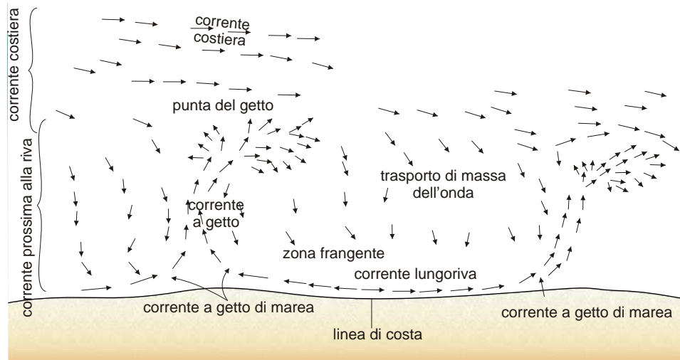
Figura 2.2.17: Modello di circolazione nella zona vicina alla spiaggia (celle di circolazione litorale):
