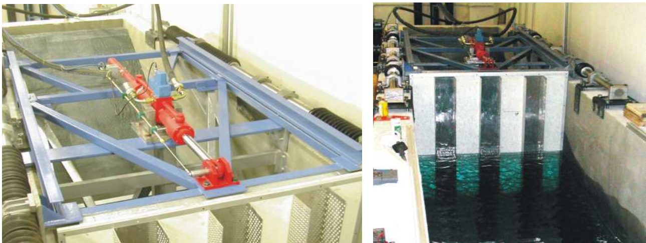
Figura 3.3.4: Pistone e pala del generatore d'onda, dal Laboratorio di Ingegneria Ambientale e Marittima dell'Università de L'Aquila.
