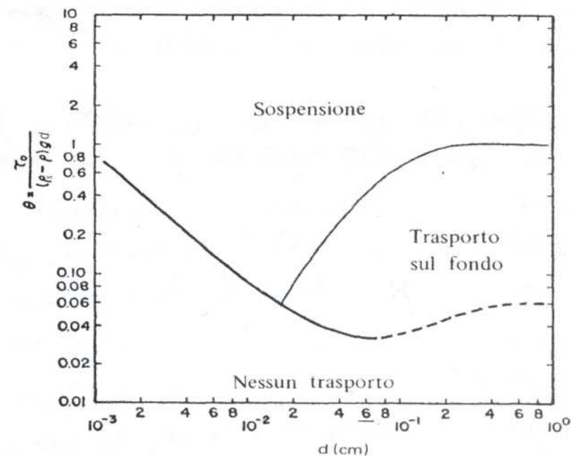
Figura 2.1.13: Diagramma di A. Shields e R.A. Bagnold. F. Ricci Lucchi, Sedimentologia parte 2
