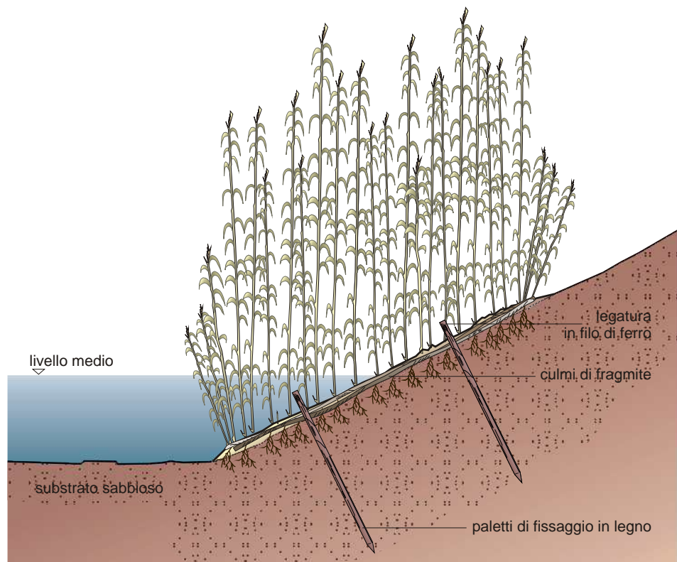
Figura 5.3.5: Copertura diffusa con culmi di canna. Si tratta di un rivestimento di sponda, precedentemente modellata, in condizioni di bassa pendenza e modesta velocità dell'acqua, con culmi di canna in numero da 30 a 60 per metro, di lunghezza da 80 a 170 cm, con la parte inferiore a contatto diretto con l'acqua (10-15 cm al di sotto del livello medio). Il fissaggio avviene mediante paletti e filo di ferro. La messa in opera potrà avvenire preferibilmente quando i giovani culmi avranno raggiunto le dimensioni necessarie (solitamente da marzo a fine maggio).
