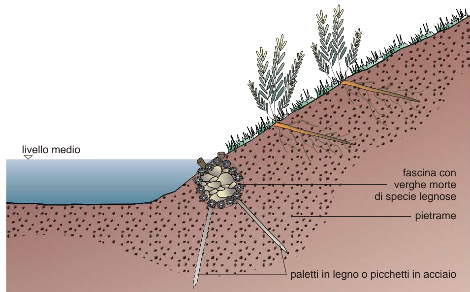
Figura 5.3.4: Fascinata sommersa. Protezione del piede della sponda mediante una fascinata costituita da legname morto di specie arbustive, caricate al centro con ghiaia o pietrisco. Viene realizzata sul posto e legata con filo di ferro, nastro metallico o tessuto sintetico, fissata con pali di legno o tondini metallici di lunghezza variabile a seconda del substrato. La tecnica, adatta per protezione di sponda nel tratto normalmente sommerso dal livello medio delle acque, va di solito abbinata con strati di ramaglia e fascine spondali vive nella parte a contatto e fuori dall'acqua.
