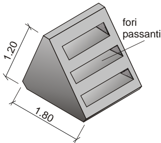
Figura 4.1.31: Elemento modulare Surgebreaker. E' utilizzato per proteggere spiagge naturali ed artificiali con provate caratteristiche di efficacia e durabilità, grazie alla sua capacità di ridurre la riflessione e l'energia ondata trasmessa.
