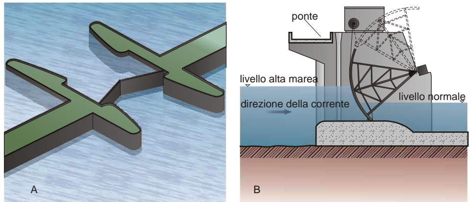
Figura 6.0.2: Esempi di barriere radiali antimarea:
