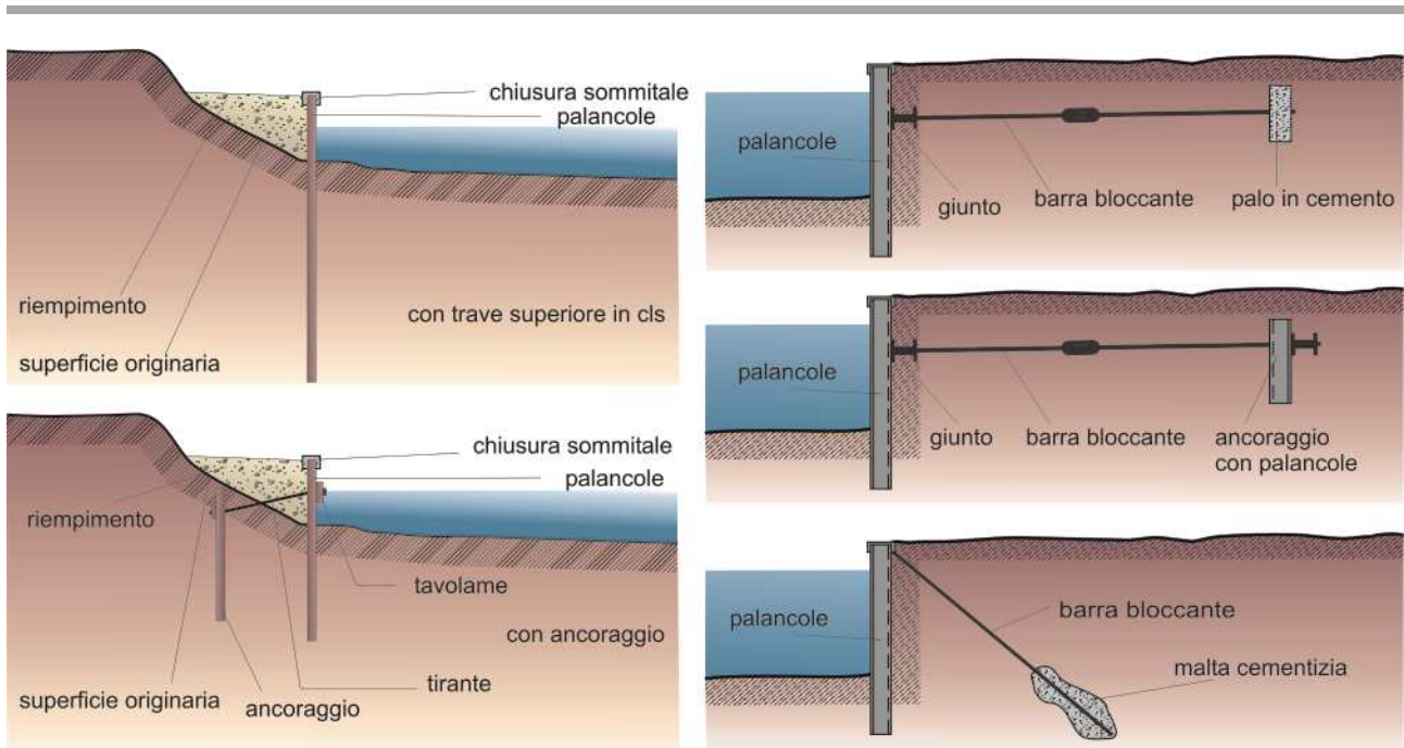
Figura 4.3.41: Sistemi di ancoraggio. I diversi tipi di ancoraggio vengono scelti in base alle caratteristiche meccaniche dei terreni e alle condizioni meteomarine locali.
