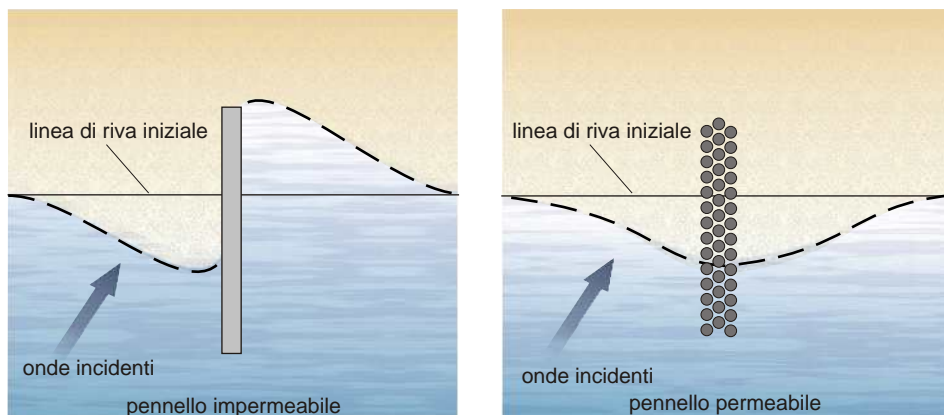
Figura 4.2.18: Pennello con palizzata in legname. L'utilizzo di una semplice struttura in legno, fa sì che grazie alla sua permeabilità non avvenga il fenomeno di dentellatura della linea di costa, con la formazione di un profilo costiero omogeneo, sia a monte che a valle dell'opera. Le strutture, una volta completate, agiscono deviando o intercettando le correnti lungo riva e, spesso, fornendo un ostacolo fisico al movimento del materiale di spiaggia. I limiti delle opere di difesa trasversali in pali di legno sono costituiti da una scarsa azione di barriera meccanica, dalla loro durata limitata e dagli alti oneri di manutenzione, nonostante il basso costo iniziale, e delle proprietà geologico-tecniche del substrato di incastro.
