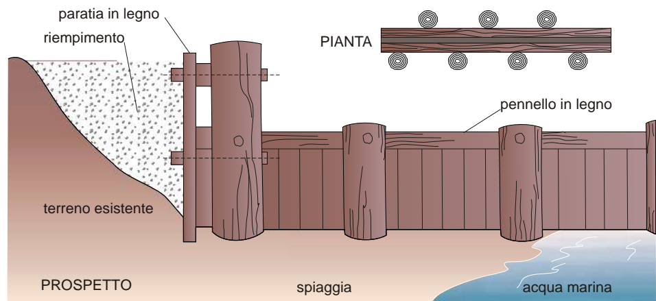
Figura 4.2.14: Pennello impermeabile con tavole e pali in legno trattati. Questo tipo di struttura è indicato per paraggi non soggetti a forte ondatazione e necessita di una buona infissione degli elementi nella sabbia e di un buon trattamento impermeabilizzante per il legname.
