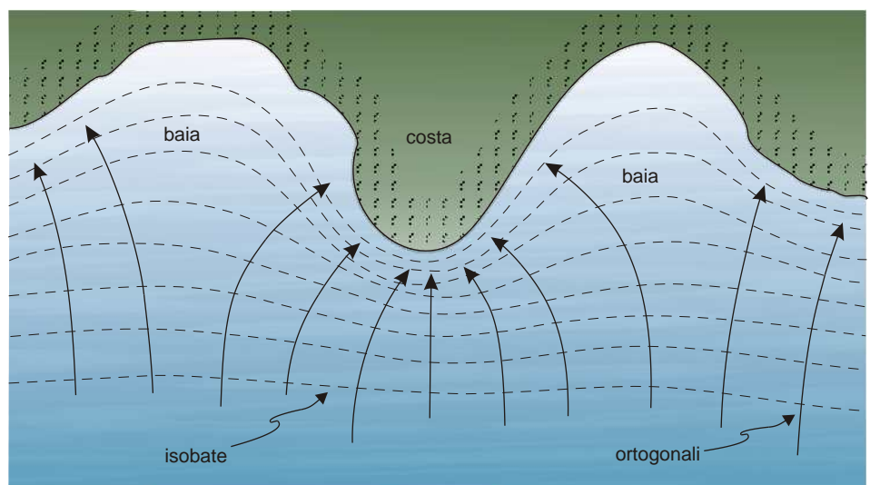
Figura 2.2.7: La spaziatura delle ortogonali d'onda (normali alle linee di cresta) è indicativa della distribuzione dell'energia del moto ondoso in prossimità della costa. Le ortogonali d'onda verso un promontorio si avvicinano tra loro, indicando una concentrazione di energia sulla costa. Verso la baia si allontanano e l'impatto delle onde risulta attenuato. Il risultato di questa distribuzione di energia è la tendenza del moto ondoso a regolarizzare le coste smantellando i promontori e colmando le insenature.
