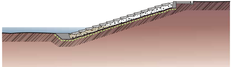
Figura 4.3.19: Rivestimento con unità Terrace Blocks. Questo sistema, oltre a favorire un'attenuazione dell'energia delle onde, consente una buona fruibilità turistico-ricreativa nel caso in cui sia presente una spiaggia antistante.
