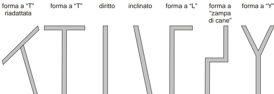
Figura 4.2.21: Possibili configurazioni dei pennelli compositi, ciascuna con caratteristiche adatte alle particolari condizioni meteomarine locali. In generale, la deposizione di sedimenti a tergo delle estremità trasversali al pennello principale favorisce una riduzione dell'altezza delle onde incidenti ed una diminuzione della pendenza della spiaggia sommersa.
