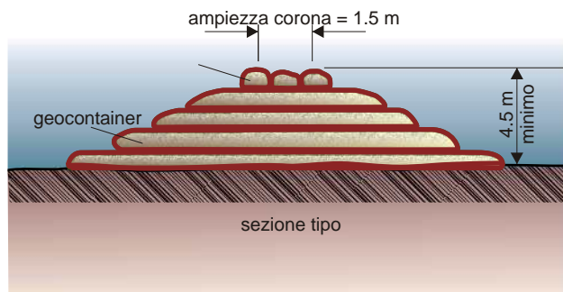
Figura 4.1.21: Barriera con Geocontainers. La struttura è simile a quella con Geotubi, ma le dimensioni degli elementi sono maggiori.
