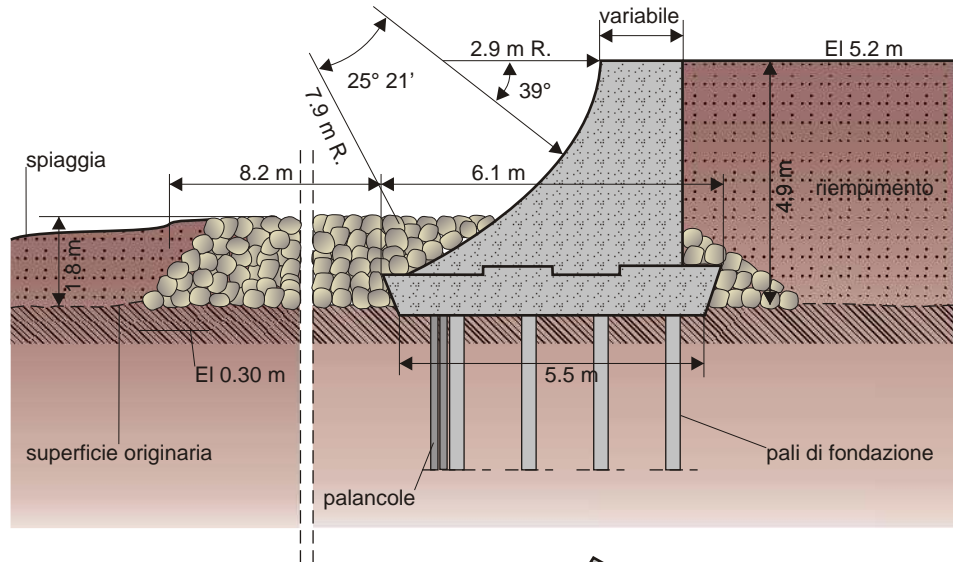
Figura 4.3.32: Esempio di realizzazione di struttura, con muro a raggio composto, fondata su pali e fronteggiata da una protezione inferiore in pietrame. La prima fila di pali viene rinforzata anteriormente grazie all'infissione di una serie di palancole.
