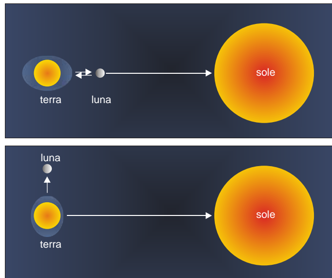
Figura 2.2.18: Le maree legate all'azione del sole amplificano o smorzano l'effetto delle maree lunari. Quando si ha luna nuova o luna piena (sole e luna allineati o in congiunzione) l'influenza dei due astri si somma: si hanno così le maggiori escursioni di marea (maree sizigiali).
