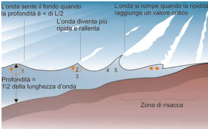
Figura 2.2.8: In prossimità della battigia l'altezza dell'onda aumenta e le creste diventano più ravvicinate.
