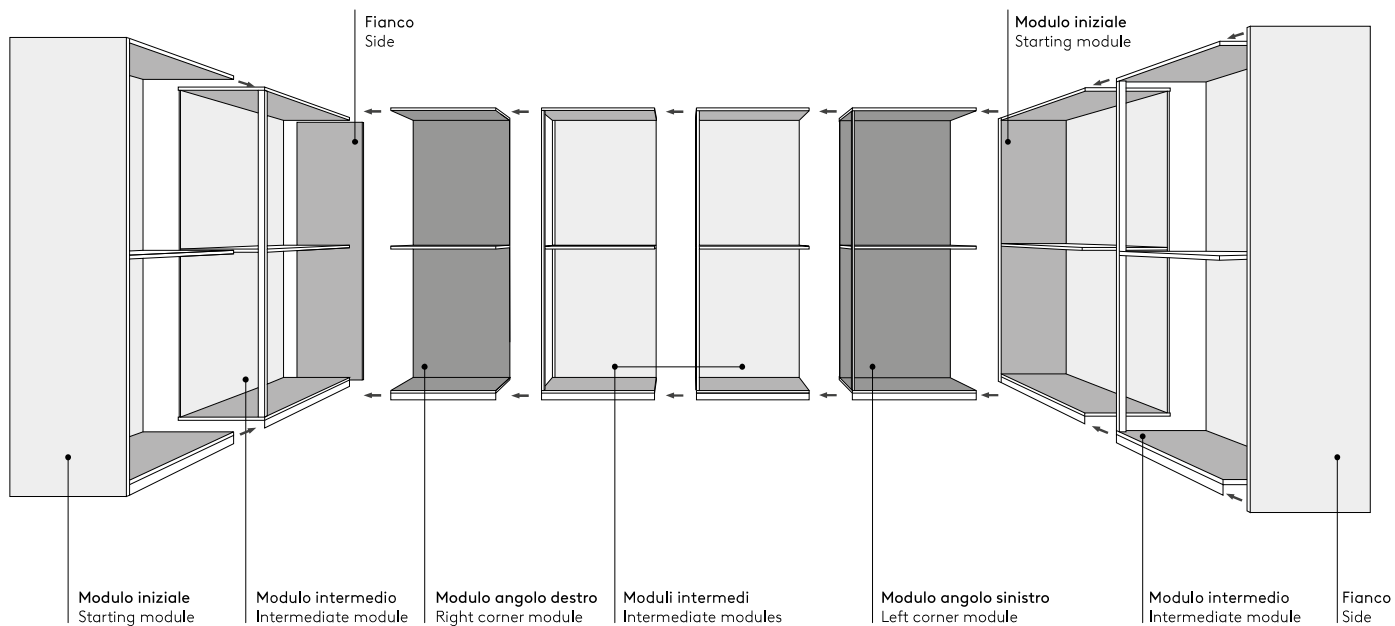
Vista esplosa Exploded view
