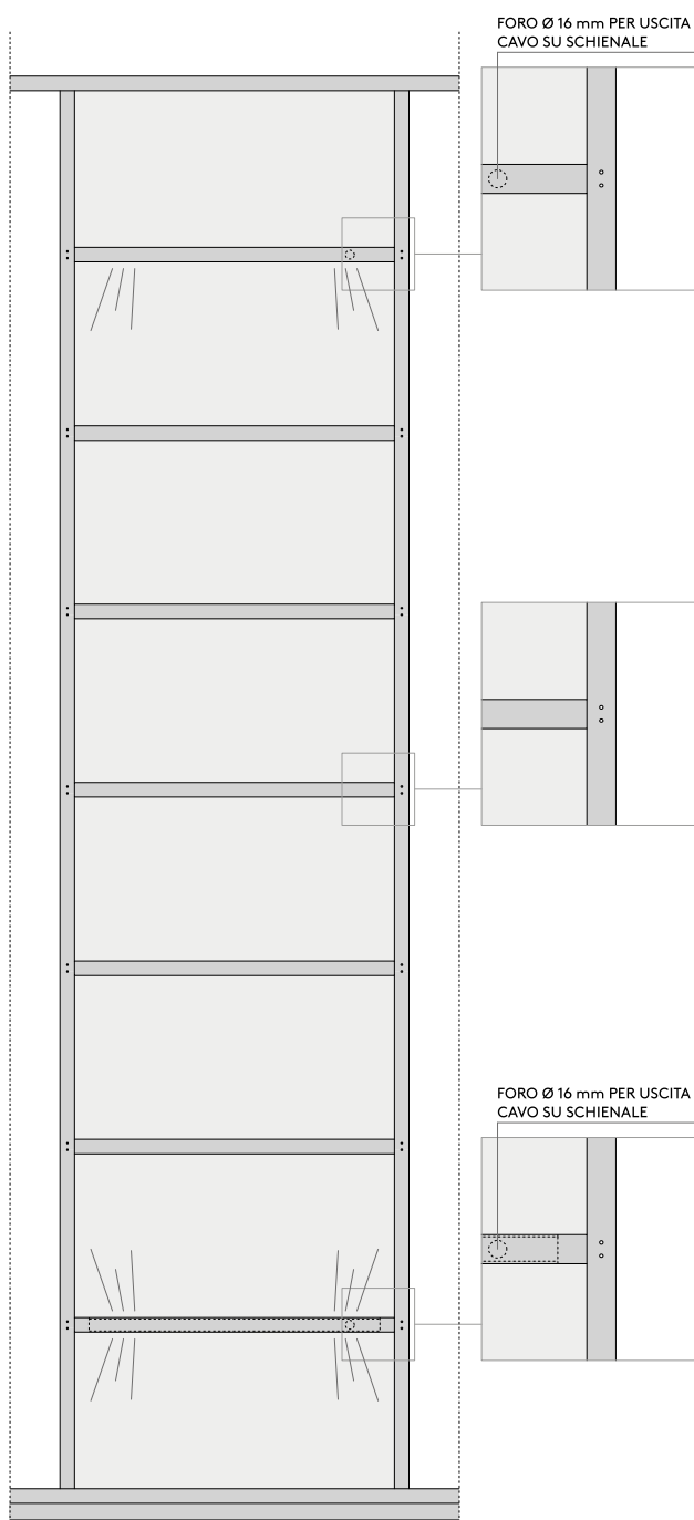
Sezione frontale Section view
