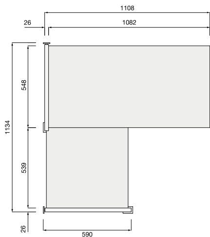
Modulo angolo LATO LUNGO DESTRO Corner module with RIGHT WIDER SIDE
