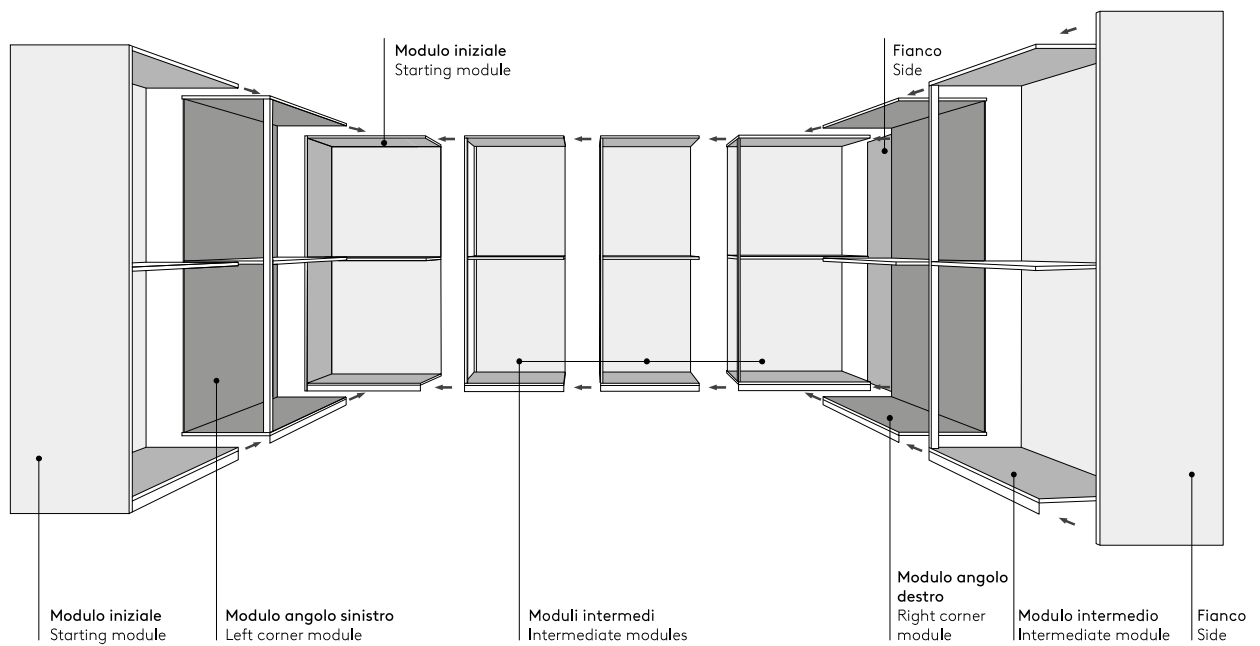
Vista esplosa Exploded view
