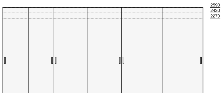
Altezze e prospetti moduli con ante Modules with doors - height and front view
