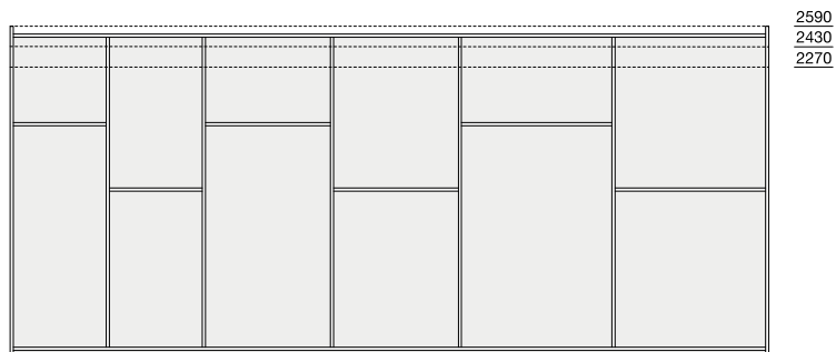
Altezze e prospetti moduli senza ante Modules without doors - height and front view
