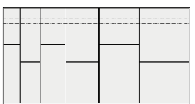
Altezze e prospetti moduli a giorno Open modules - height and front view
