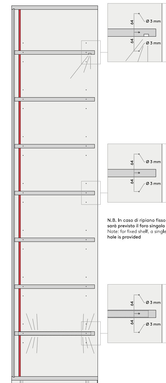
Sezione laterale Section view
