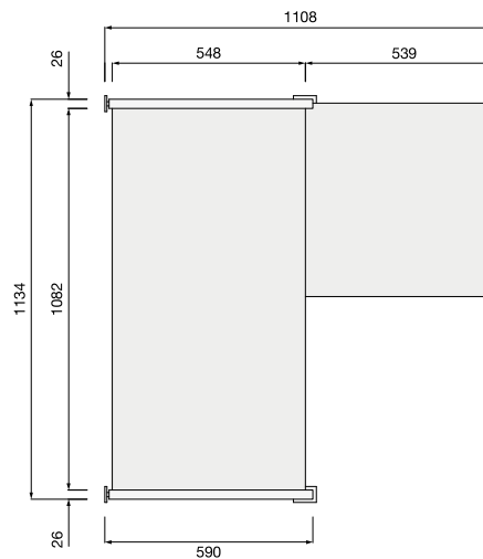
Modulo angolo LATO LUNGO SINISTRO Corner module with LEFT WIDER SIDE
