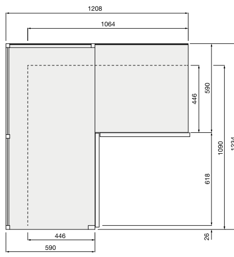
Con montante e fondali legno With upright and wooden back panels
