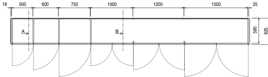
Larghezze moduli fianco legno/montante interno Width of the modules with wooden side/internal upright
