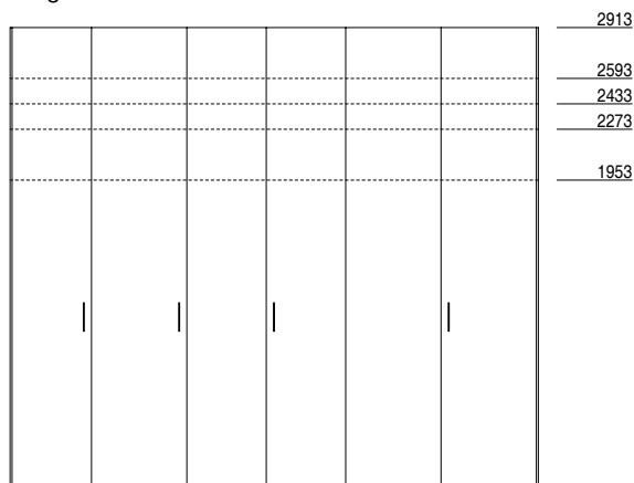
Altezze moduli con ante Height of the modules with doors
