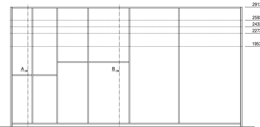
Altezze moduli senza ante Height of the modules without doors
