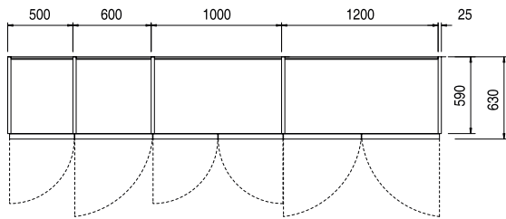
Larghezze moduli fianco legno Width of the modules with wooden side
