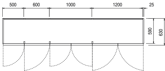
Larghezze moduli montante interno Width of the modules with internal upright
