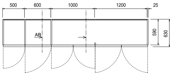
Larghezze moduli fianco legno/montante interno Width of the modules with wooden side/internal upright
