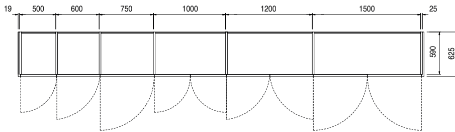
Larghezze moduli fianco legno Width of the modules with wooden side
