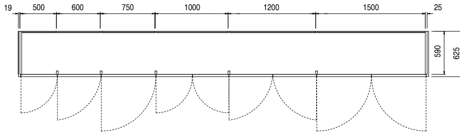
Larghezze moduli montante interno Width of the modules with internal upright
