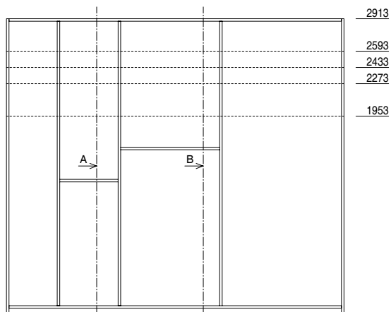
Altezze moduli senza ante Height of the modules without doors
