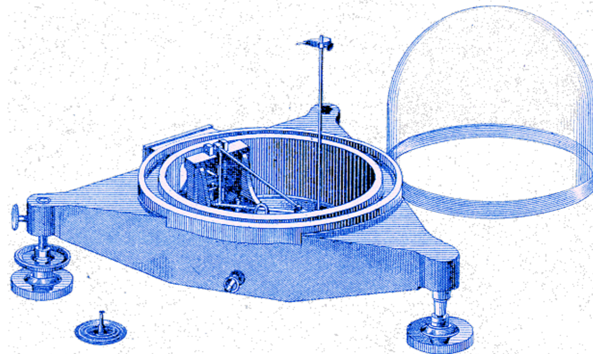
The horizontal pendulum of von Rebeur Paschwitz
