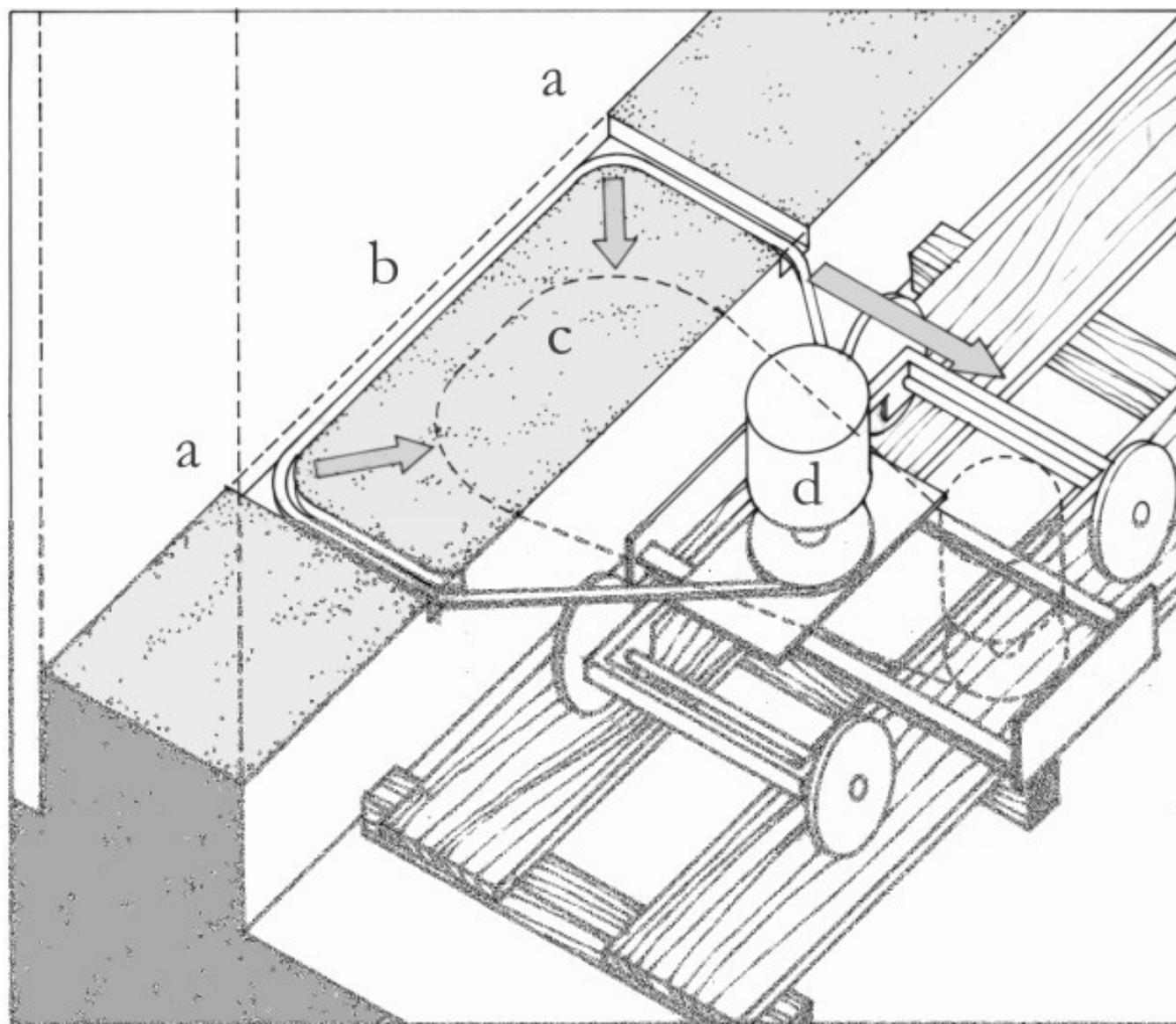
Figura 4 • Taglio meccanico della muratura con filo a sferette di acciaio diamantato: a) fori iniziali per l'introduzione del filo; b) posizione del filo all'inizio dell'operazione di taglio; c) posizione del filo a operazione avanzata; d) puleggia motrice.
