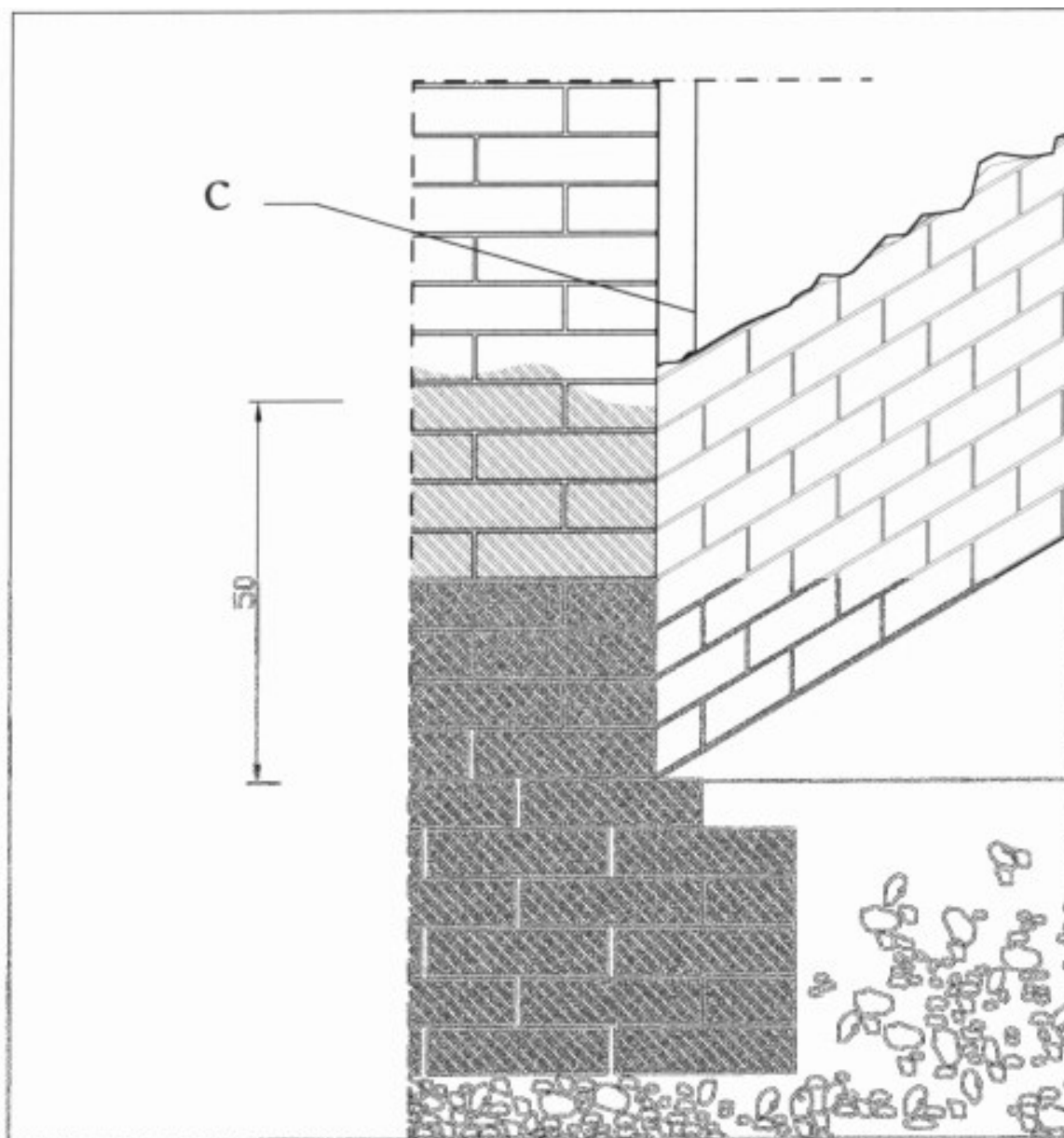
Figura 2 • Schema del sistema di intercettazione capillare. Rimozione dell'intonaco per almeno 30 cm oltre il livello raggiunto dall'umidità di risalita. c) Rimozione dell'intonaco.
