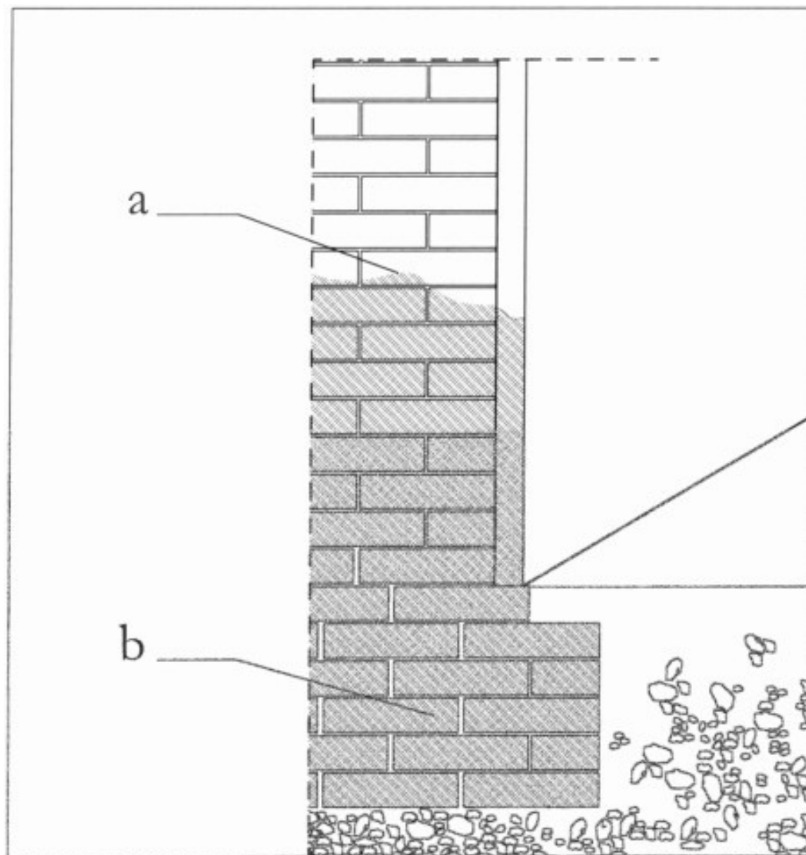
Figura 1 • Schema del sistema di intercettazione capillare. Muratura soggetta a umidità di risalita capillare. a) Livello di risalita capillare; b) fondazione umida.
