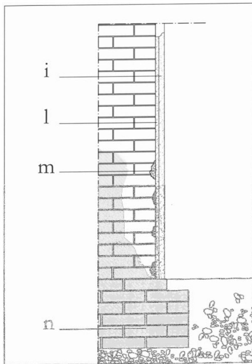
Figura 4 • Applicazione di intonaco macroporoso. Dopo almeno 24-48 ore, a rinzafo ben indurito, previa bagnatura, si procede nell'applicare il successivo strato di intonaco di spessore variabile tra 2 e 4 cm. i) Intonaco macroporoso; l) rinzafo; m) integrazioni; n) fondazione umida.
