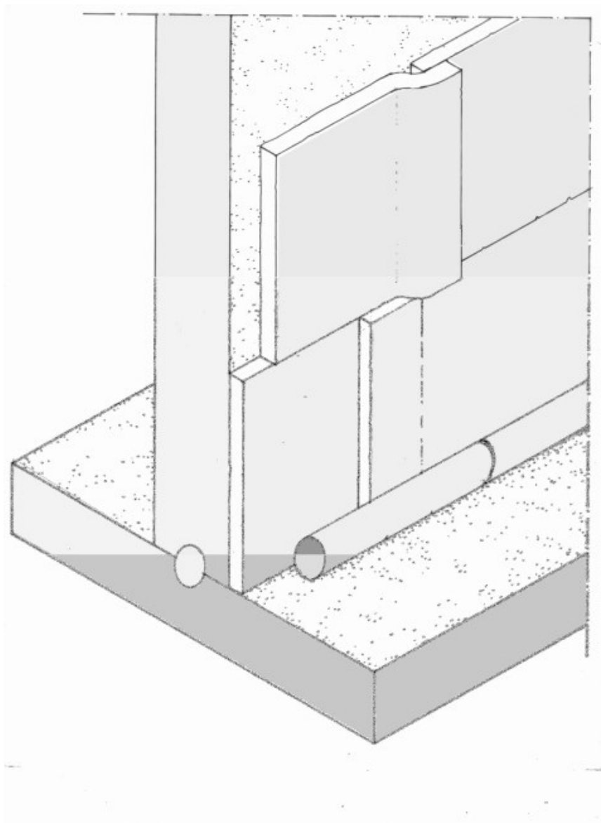
Figura 1 • Protezione delle fondazioni con pannelli di bentonite di sodio. Applicazione sulla faccia verticale di pannelli di dimensioni 50 x 60. Nel punto di contatto tra piano verticale e piano orizzontale è posato un cilindro dello stesso materiale per evitare eventuali possibili infiltrazioni di acqua proveniente dal terreno.
