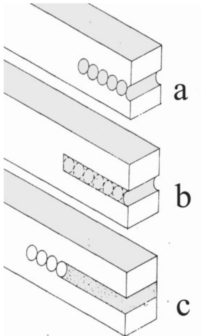
Figura 6 • Fasi di realizzazione del taglio con carotatrice: a) prima serie di fori; b) seconda serie di fori sovrapposti a quelli precedenti, in modo da asportare le parti di muratura rimaste; c) il primo varco è riempito di resina poliester. A presa avvenuta, senza bisogno di zeppe, si può procedere al taglio del tratto adiacente.
