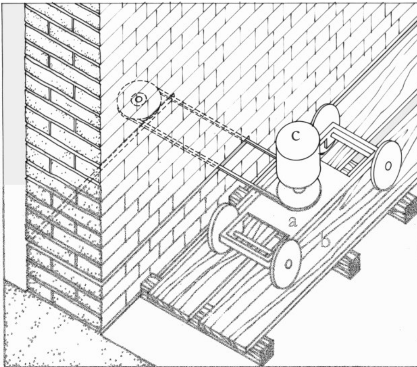
Figura 3 • Taglio meccanico della muratura con sega a catena: a) carrello porta sega; b) palanche appoggiate sul terreno per consentire lo scorrimento orizzontale del carrello; c) sega a catena.
