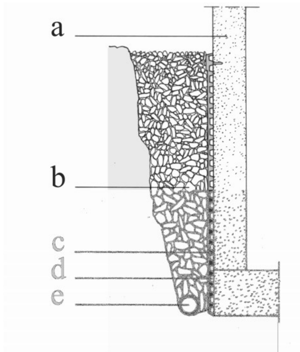
Figura 2 • Protezione delle fondazioni con membrana in polietilene. I pannelli dell'altezza dell'intera porzione di muro da proteggere sono fissati alle pareti mediante viti a espansione.
