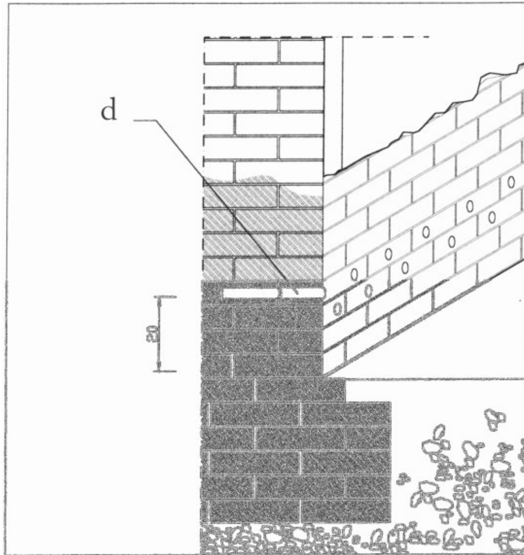
Figura 3 • Schema di applicazione di intercettazione capillare.
