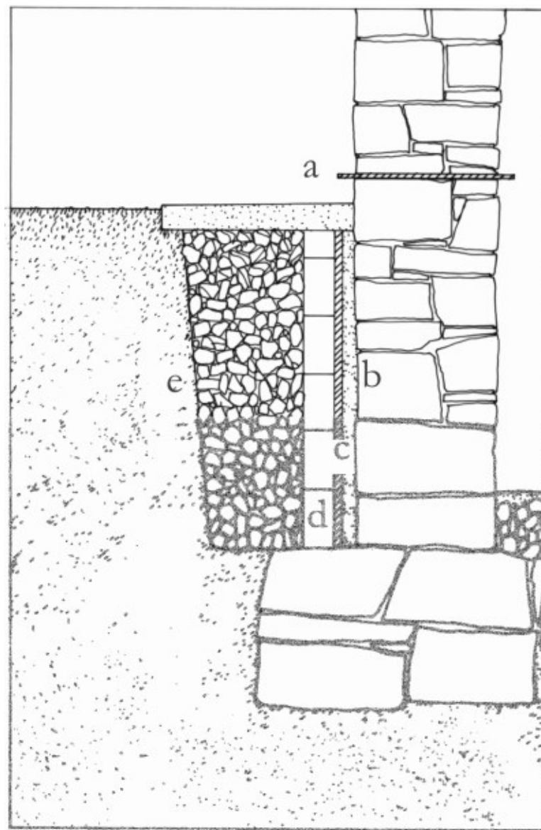
Figura 2 • Schema di una fossa drenante aderente al muro. a) barriera orizzontale impermeabile; b) intonaco; c) eventuale impermeabilizzazione; d) muretto di mattoni posti in opera a coltello; e) riempimento in pietrame.
