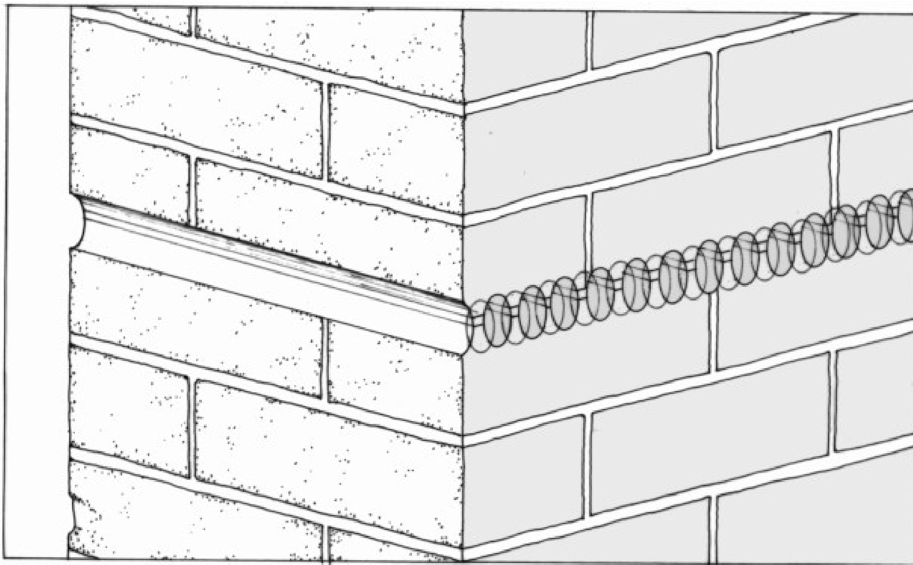
Figura 5 • Il metodo Massari consiste nell' eseguire il taglio meccanico delle murature utilizzando una carotatrice. Questo strumento, oltre a ridurre al minimo urti e vibrazioni, consente, grazie al suo moto rotatorio uniforme, di perforare muri di notevole spessore.
