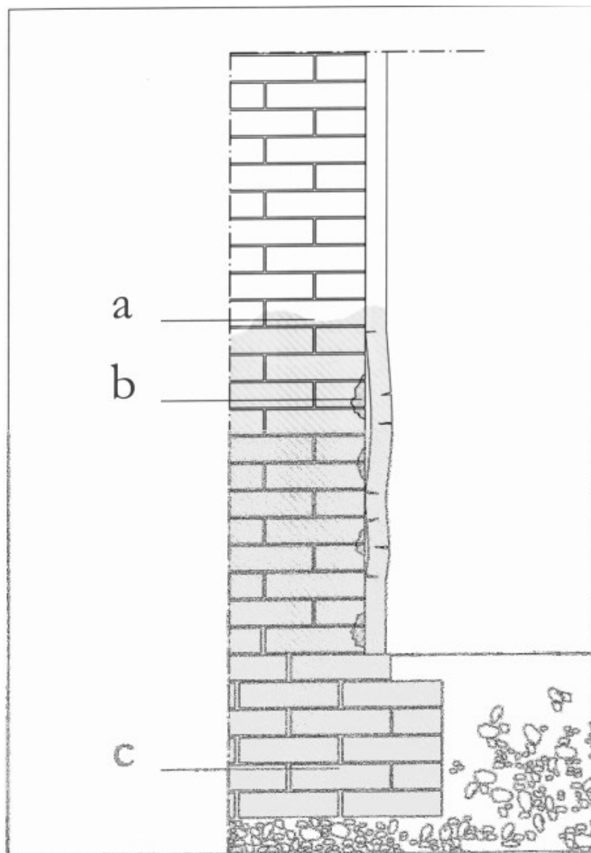
Figura 1 • Muratura soggetta a umidità di risalita capillare. a) Livello di risalita capillare; b) porzioni di muratura spugnosa o friabile; c) fondazione umida.
