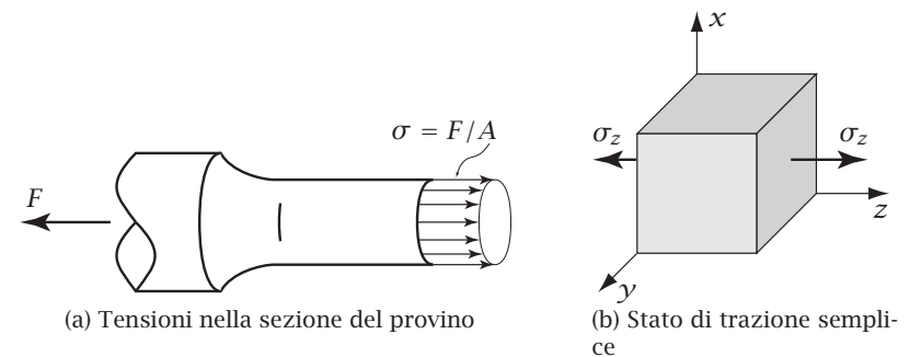
Figura 4.2: Tensioni nella prova di trazione
