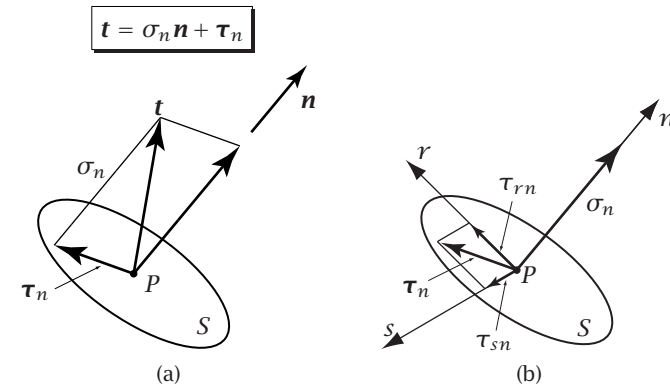
Figura 3.12: Componente normale e componente tangenziale
