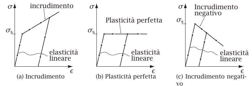
Figura 4.9: Elastoplasticità bilatera
