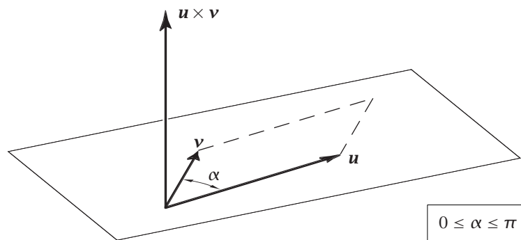
Figura 1.2: Prodotto vettoriale
