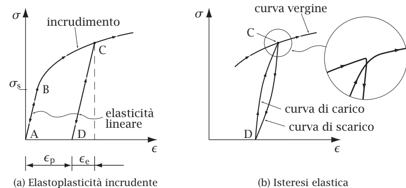
Figura 4.8: Elastoplasticità
