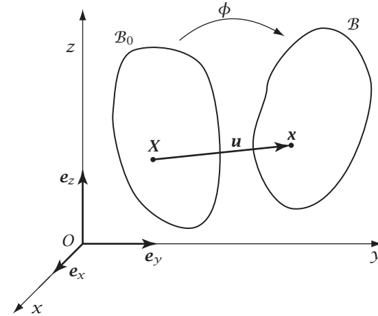
Figura 3.2: Deformazione e spostamento
