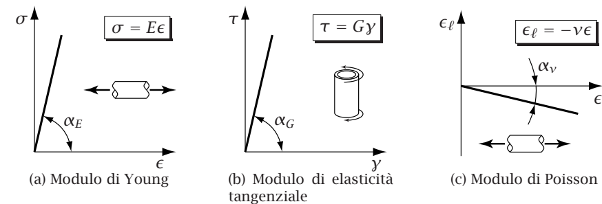
Figura 4.6: Elasticità lineare
