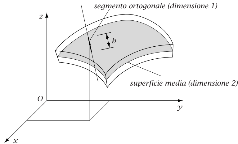
Figura 2.10: Lastra (modello bidimensionale con struttura)
