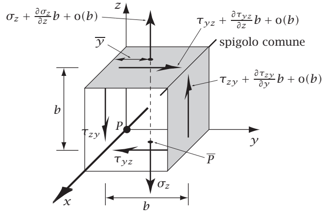
Figura 3.15: Dimostrazione della reciprocità delle tensioni tangenziali
