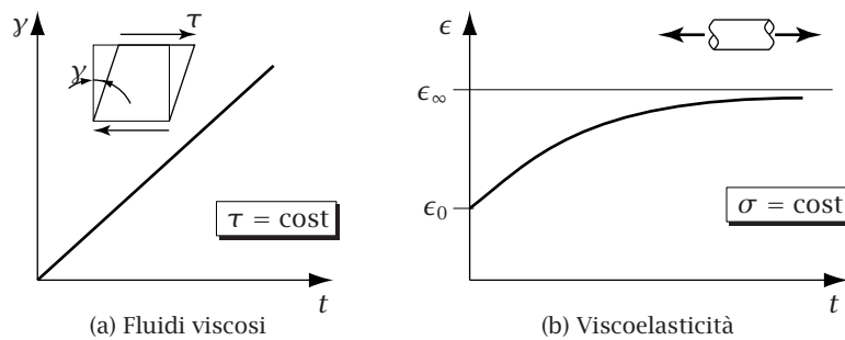
Figura 4.10: Viscosità
