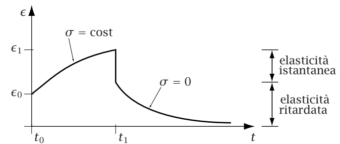
Figura 4.11: Elasticità ritardata
