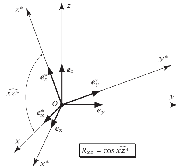
Figura 1.9: Componenti di una rotazione
