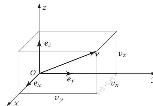
Figura 1.6: Decomposizione di un vettore
