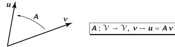
Figura 1.4: Tensore doppio
