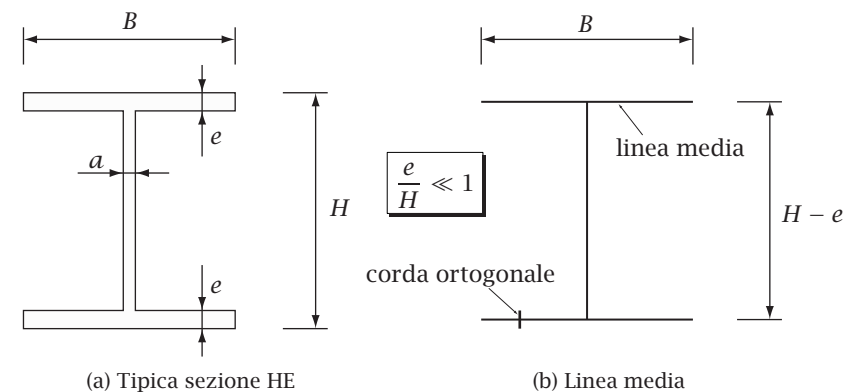
Figura 2.6: Sezione sottile aperta
