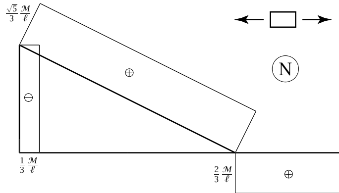
(a) Forza normale
