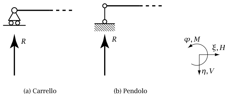
Figura 1.7: Vincoli che impediscono l'incremento di spostamento in una data direzione
