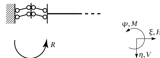
Figura 1.8: Doppio doppio pendolo (pendolo improprio)
