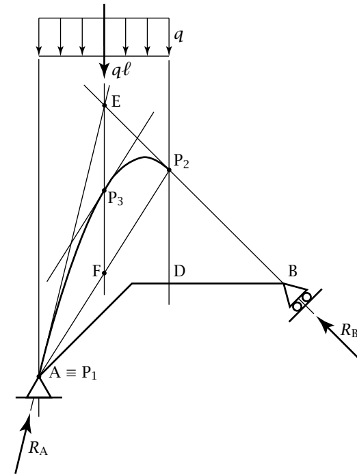
Figura 3.8: Costruzione della curva delle pressioni parabolica
