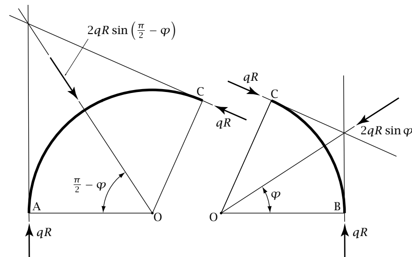
Figura 3.11: Reazioni interne ed esterne
