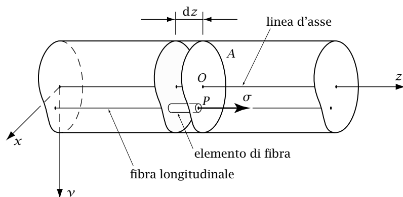
Figura 5.1: Generica fibra longitudinale
