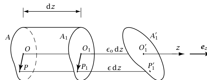
Figura 5.5: Dilatazione delle fibre longitudinali
