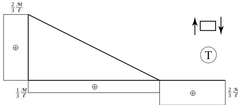
(b) Taglio
