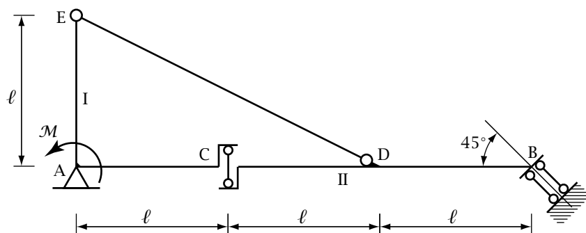
Figura 3.13: Sistema di travi chiuso soggetto ad una coppia
