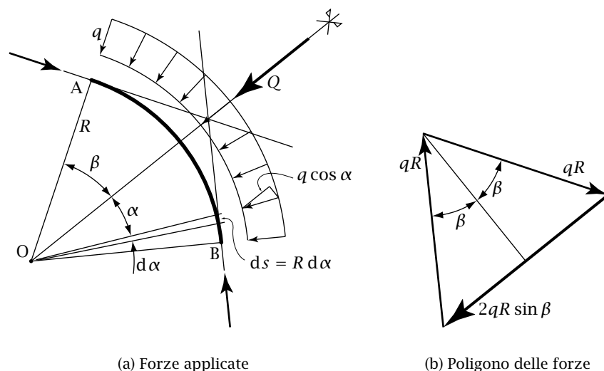
Figura 3.9: Equilibrio di un arco circolare soggetto ad un carico radiale
