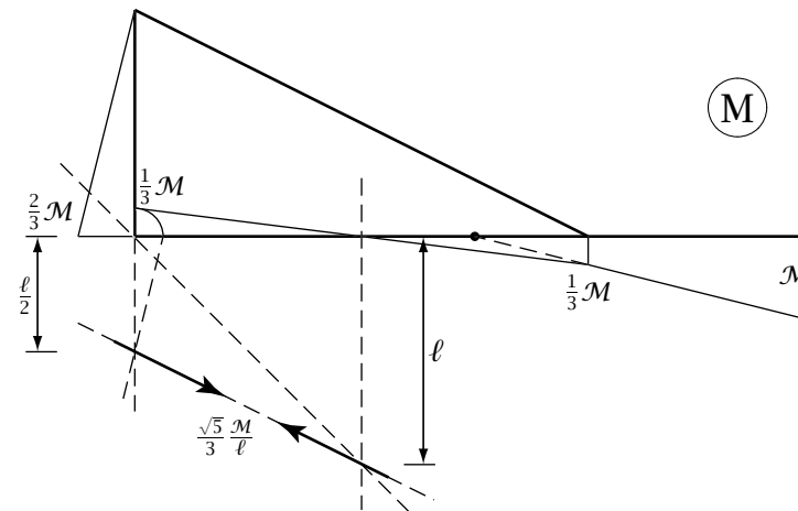
Figura 3.16: Diagramma del momento flettente
