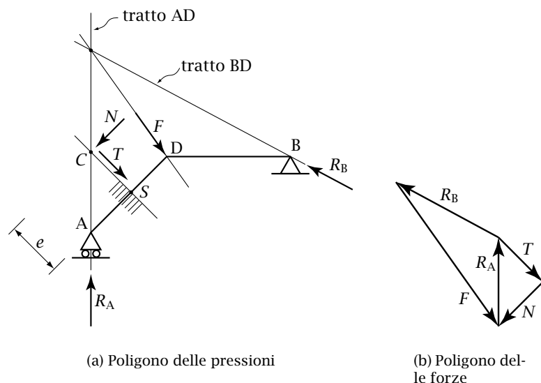
Figura 3.5: Esempio di un sistema di travi soggetto ad un carico concentrato
