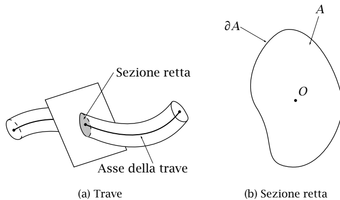
Figura 1.1: Geometria della trave
