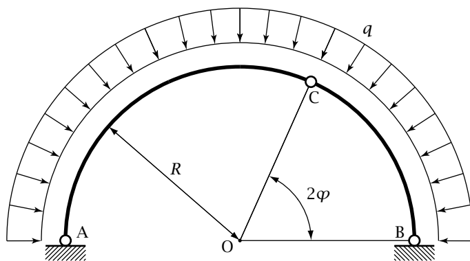
Figura 3.10: Arco circolare a tre cerniere soggetto ad un carico ripartito radiale
