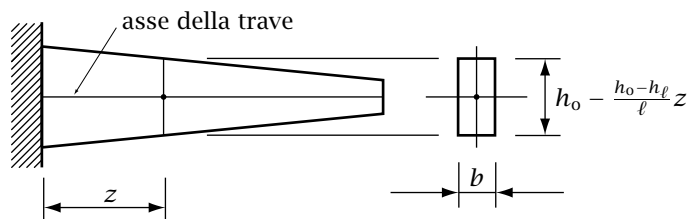
Figura 1.4: Modello geometrico della mensola
