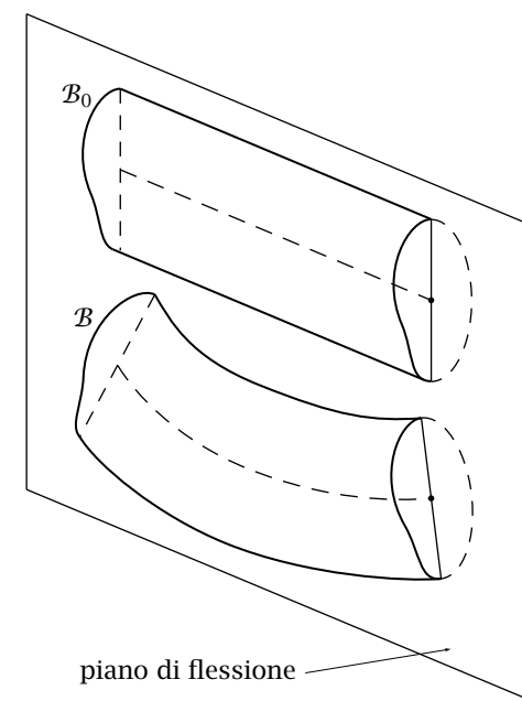
Figura 1.6: Trave cinematicamente piana
