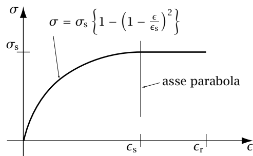
Figura 5.4: Calcestruzzo compresso
