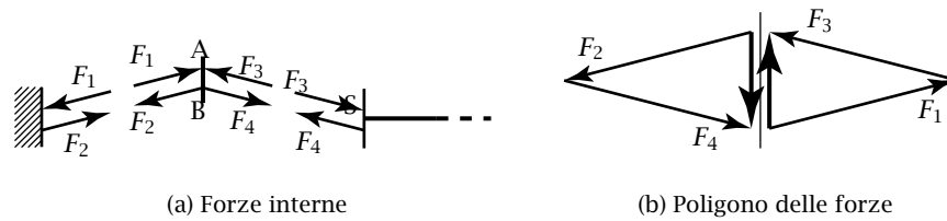
Figura 1.9: Equilibrio interno al doppio pendolo
