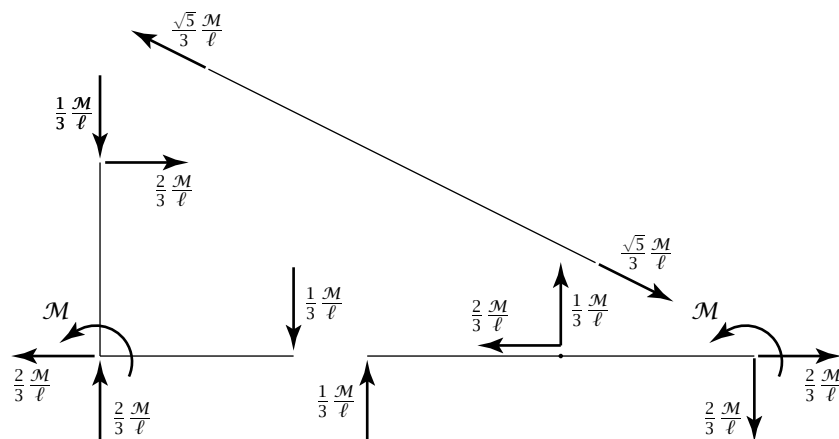
Figura 3.15: Reazioni interne ed esterne
