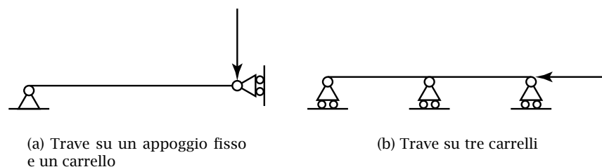
Figura 3.4: Esempi di travi labili non equilibrate
