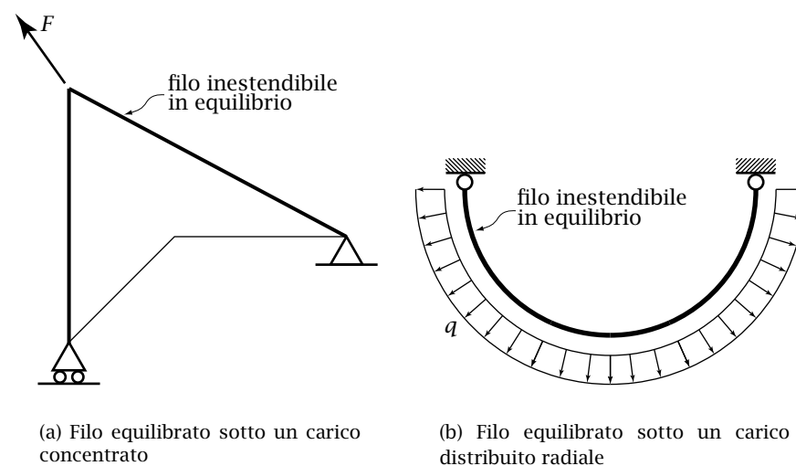
Figura 3.12: Fili inestendibili in equilibrio
