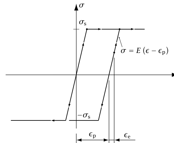
Figura 5.3: Elastoplasticità
