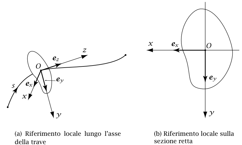
Figura 1.2: Riferimento locale
