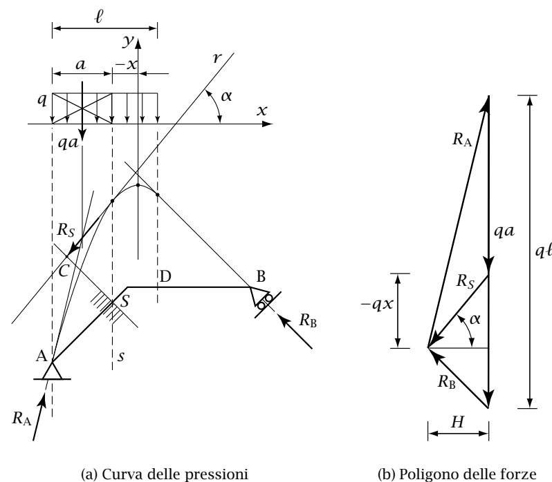
Figura 3.6: Esempio di un sistema di travi soggetto ad un carico ripartito
