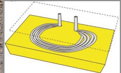
Pramollichnus pastae
