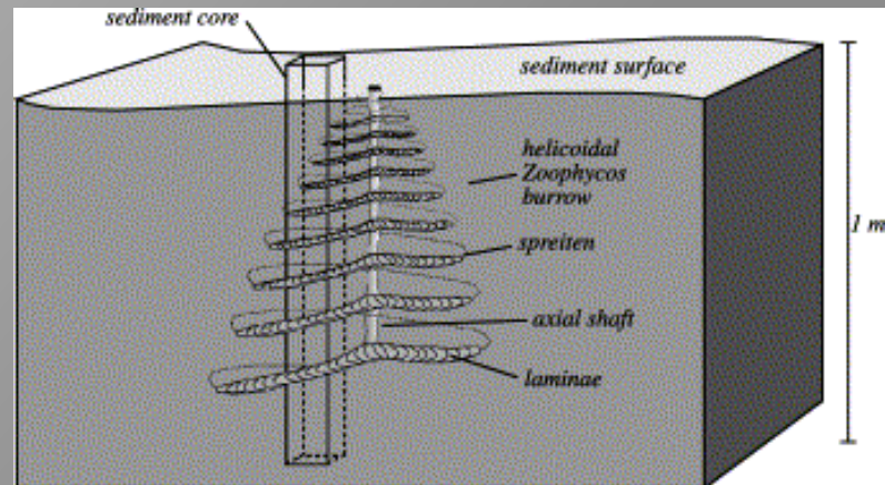
Zoophycos
