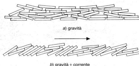
Fig. 2.15 - Orientazione spaziale (in sezione) di elementi discoidali depositati sotto il controllo della sola gravità (a) e della gravità più una corrente unidirezionale (b). In questo secondo caso i ciottoli risultano embriicati (si veda anche fig. 2.17). (Ridisegnato da Potter e Pettijohn, 1963.)
