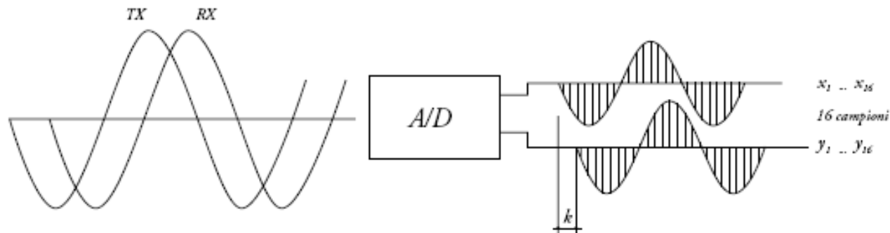
Fig. 11.5 – Trasformazione analogico-digitale e campionamento.
