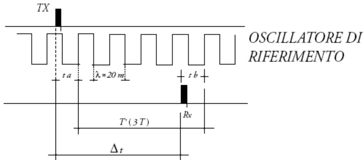
Fig. 11.6 – Metodo di invio degli «impulsi».
