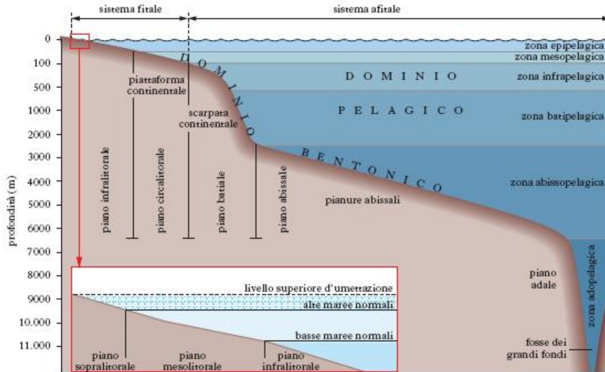
BENTONOS – Le principali suddivisioni orizzontali e verticali degli ambienti marini bentonici; nel riquadro in basso a sinistra è schematizzata la zona di marea. Per esigenze di rappresentazione, la scala delle profondità non è lineare (figura ridisegnata da B. Baccetti e altri, Zoologia. Trattato italiano , I, Bologna 1995)
