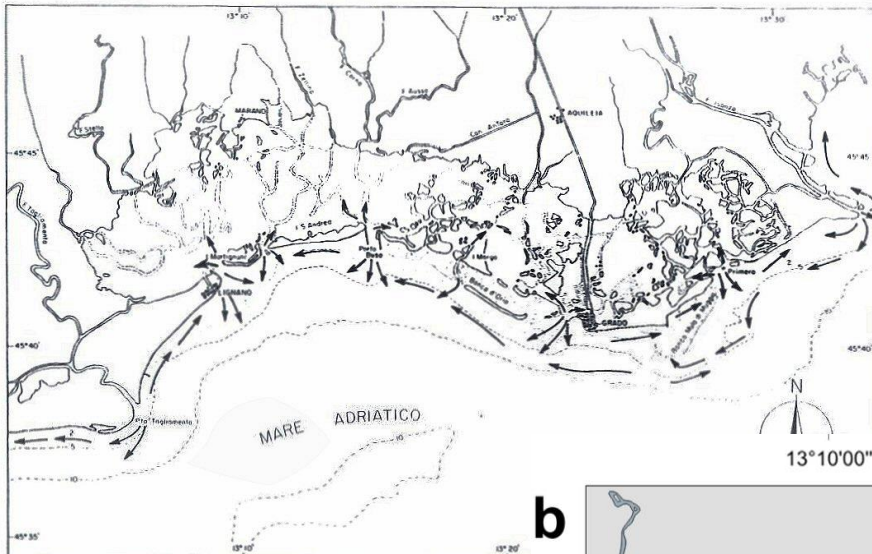
Fig. 16 - In corrispondenza delle foci lagunari il trasporto lungo riva è interrotto
