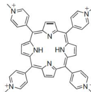
TmPyP4
