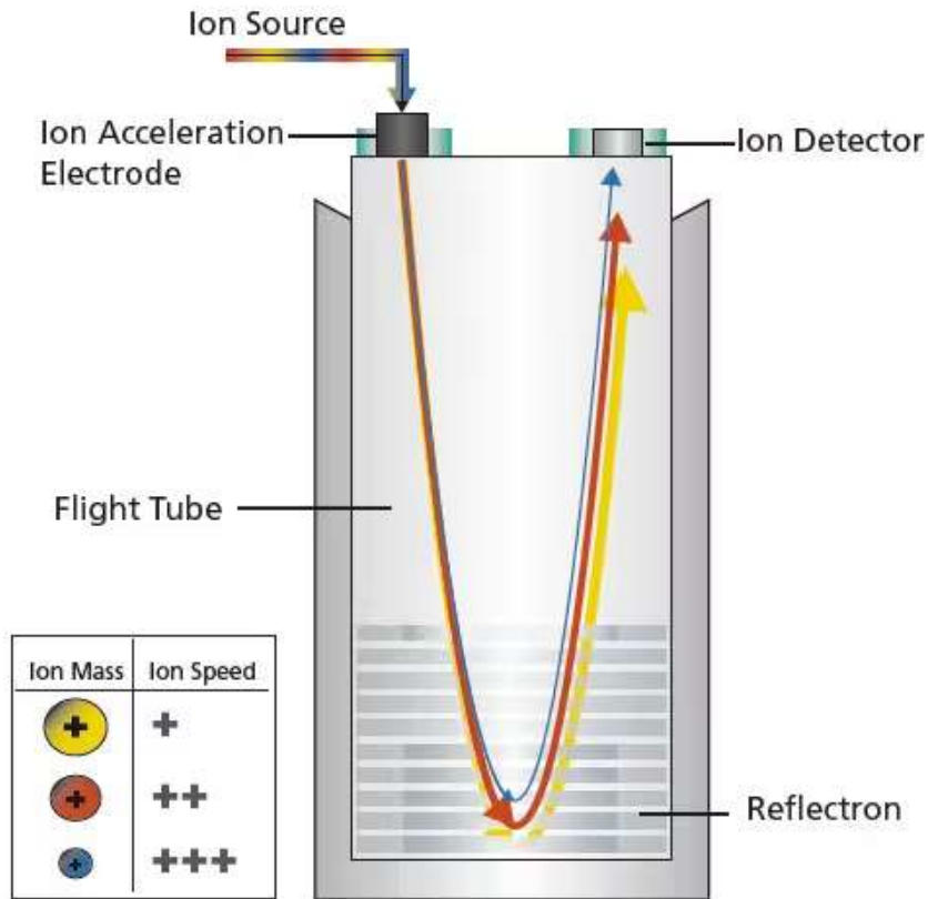
Analizzatore Time-of-Flight (TOF)
