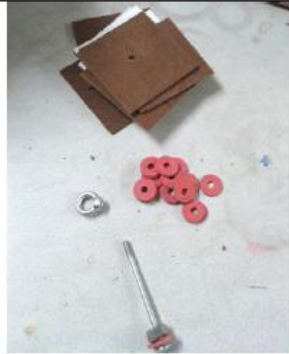
Fig.10: materiale per i SA: lamelle di faesite grezza, un perno, guarnizioni di stanziatrici di gomma e un golfaro
