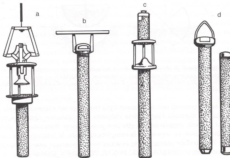
Fig. 27 - Vari tipi di carotatori: a) modello autoregolantesi con tubo acrilico (mod. R.I.C.), b) modello ad uso manuale (per basse profondità), c) modello regolato mediante caduta del messaggero, d) modello a gravità con base rastremata.
