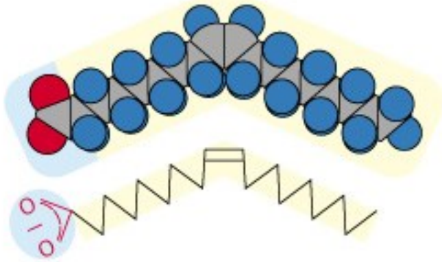
(b) Oleate ion
