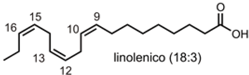
Acido \alpha -linolenico 18:3 \Delta^{9,12,15} oppure 18:3 \omega 3
