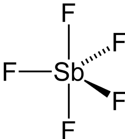
Geometria bipiramidale trigonale
