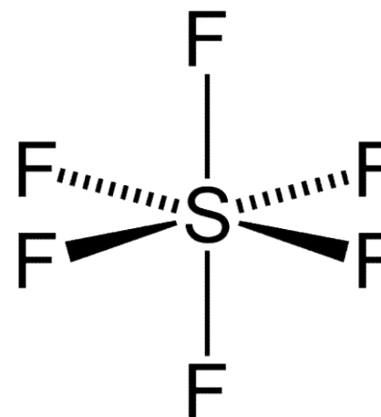
Geometria ottaedrica
