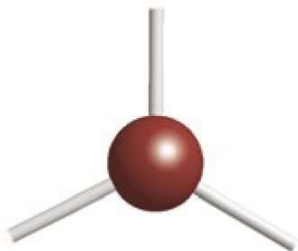
Triangolare planare
