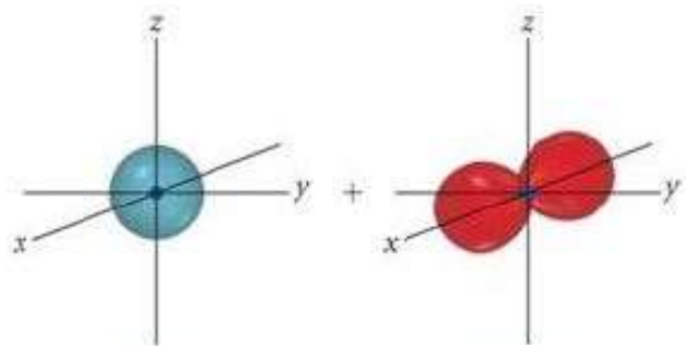
Orbitale s
