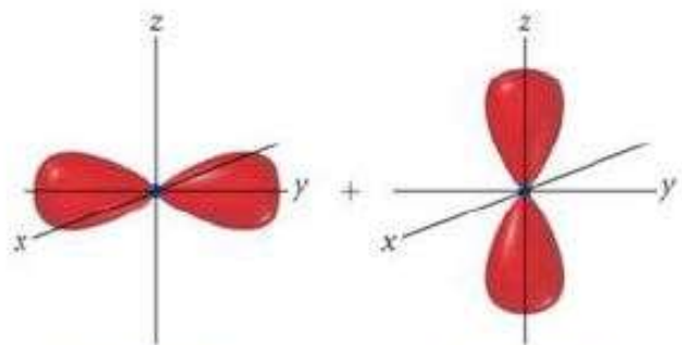
Orbitale p_y
