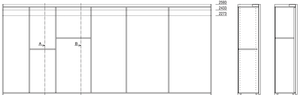
Altezze moduli senza ante Height of the modules without doors
