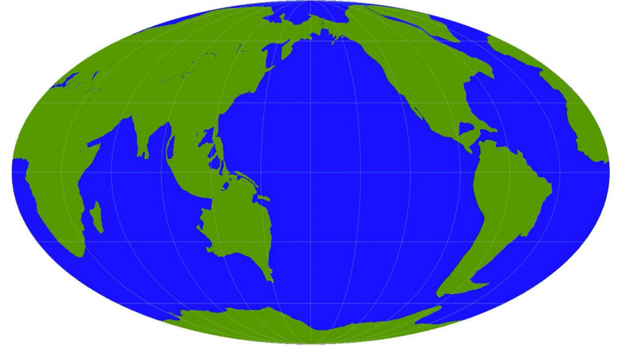
Novopangea
