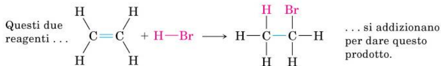
Etilene (alchene)
