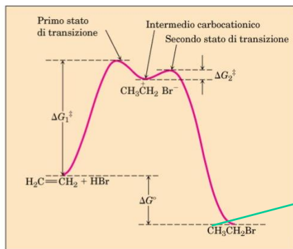
Etilene (alchene)
