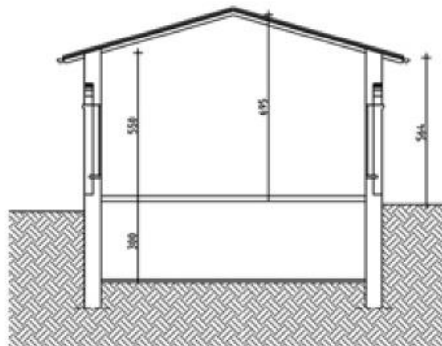
SEZIONE B-B
