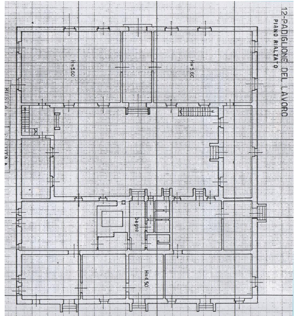
Planimetria catastale, s.d. ma >1939 <2016 (secondo impianto)
