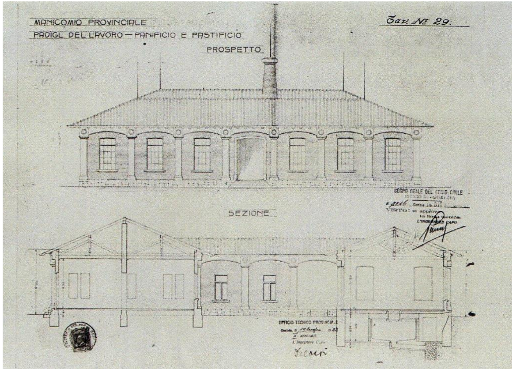
Progetto esecutivo, datato 1931, approvato nel 1932 (secondo impianto)
