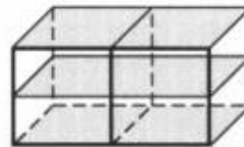
(002)
