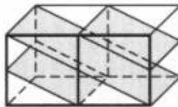
(0 \bar{1}2 )
