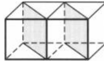
( \bar{1}\bar{1}0 )
