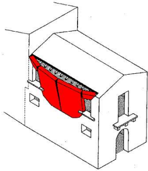
Flessione orizzontale fuori piano
