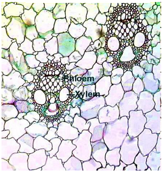
Fascio vascolare
