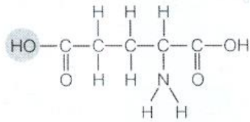
Acido glutammico Aminoacido
