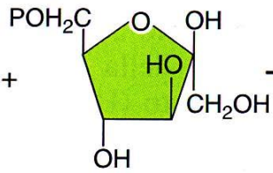
Fruttosio 6-fosfato
