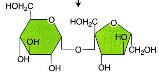
Saccarosio
