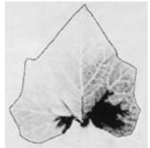
50% espansione
