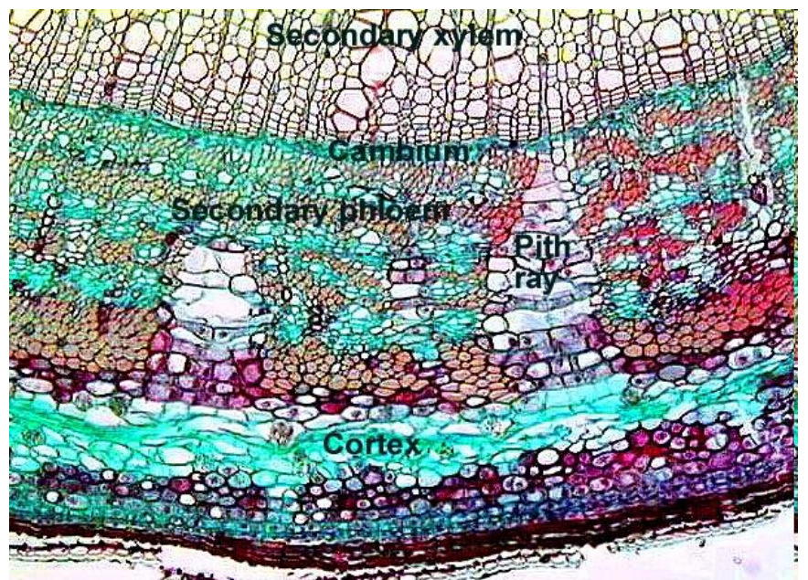
Fusto, struttura secondaria
