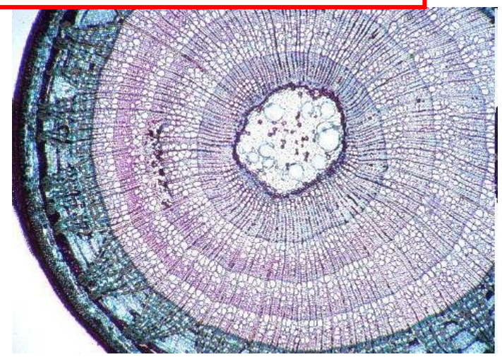
Fusto, struttura secondaria
