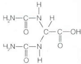
Acido allantoico
