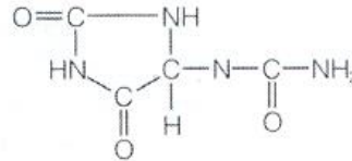
Allantoina
