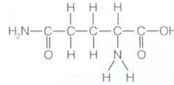
Glutammina Ammide
