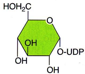
UDP-glucosio
