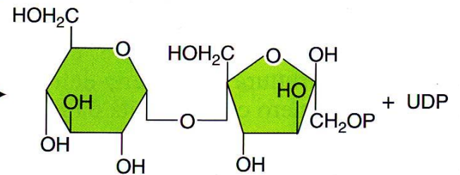
Saccarosio-6 F -fosfato
