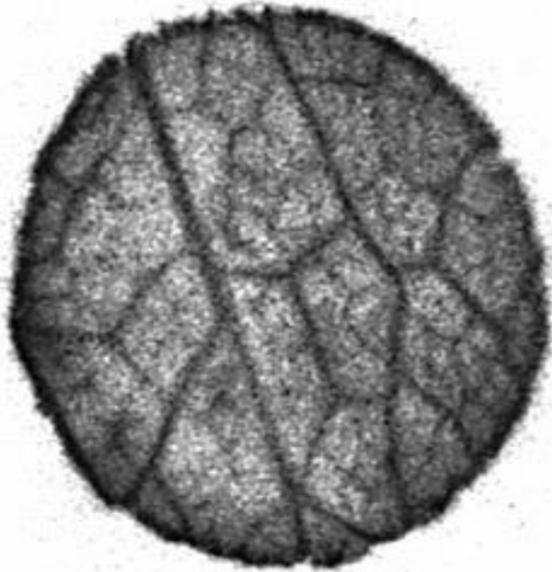
Caricamento apoplastico
