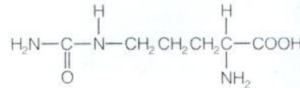
Citrullina
