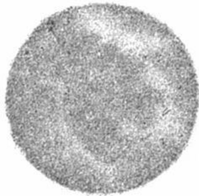
Caricamento simplastico
