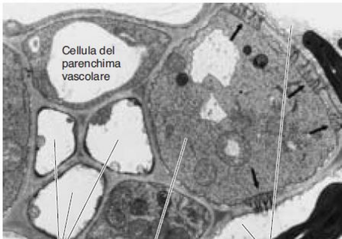
Elementi del cribro
