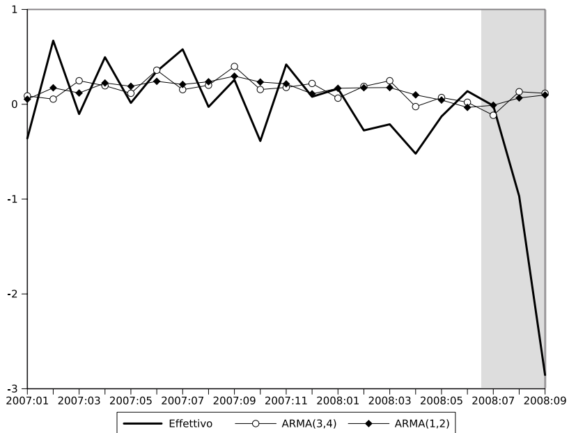
Figura 2.15: Previsioni
