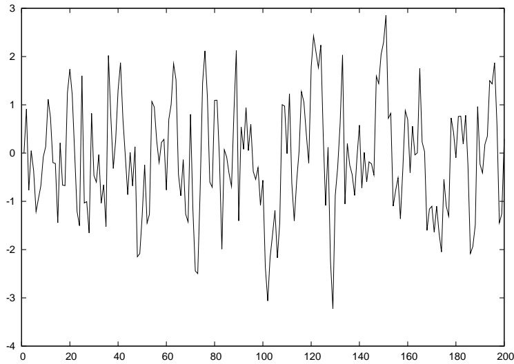
Figura 2.6: AR(1): \varphi = 0.5
