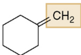
Metilenecicloesano
