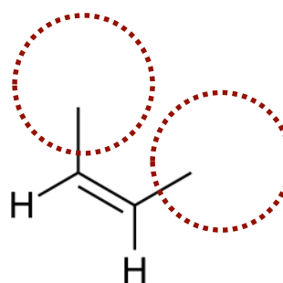
cis
