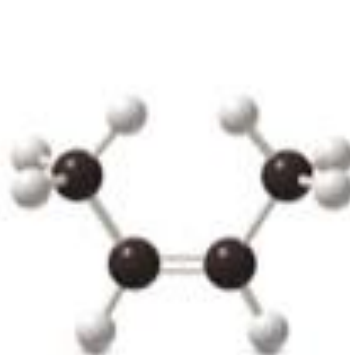
cis -2-butene
