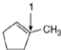
1-metilciclopentene
