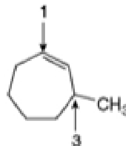
3-metilcicloeptene
