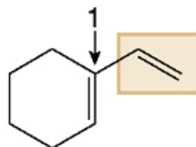
1-vinilcicloesene
