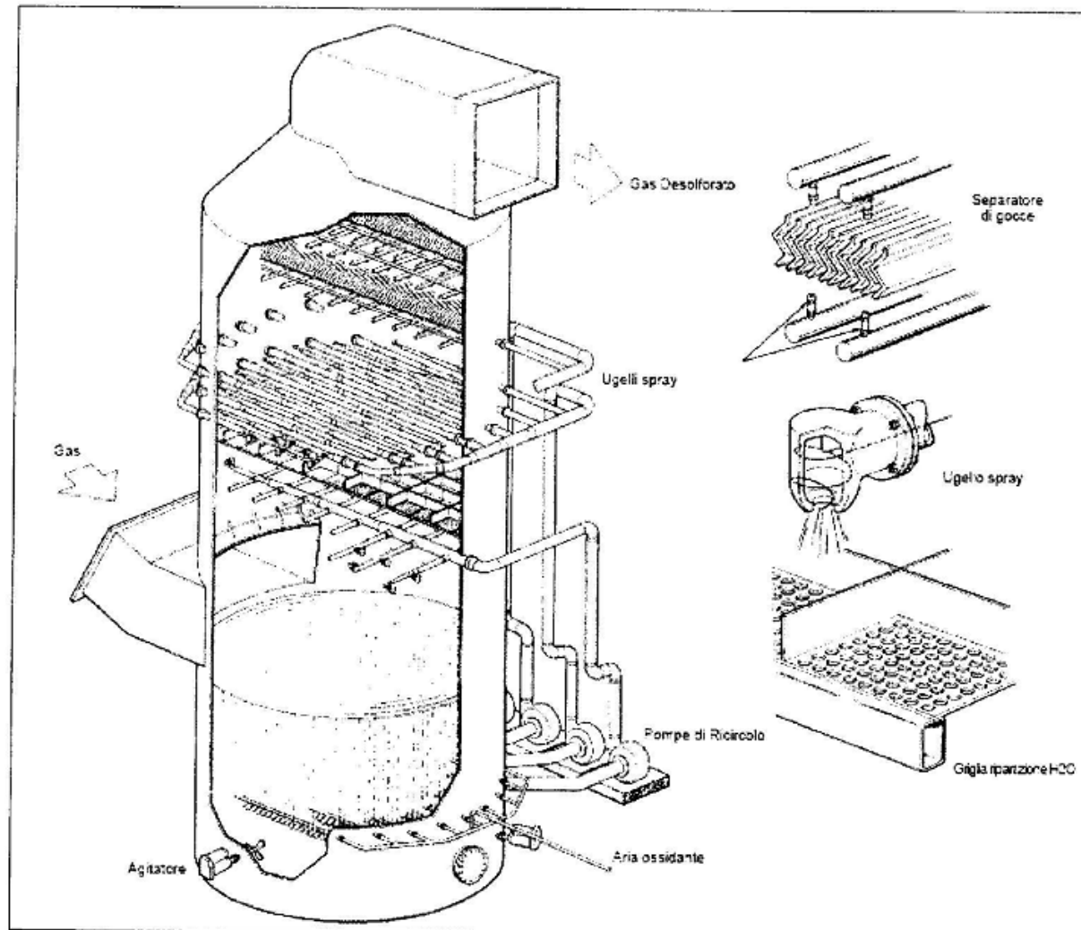
Fig.A4.16: Schema di un sistema 'wet scrubber'.
