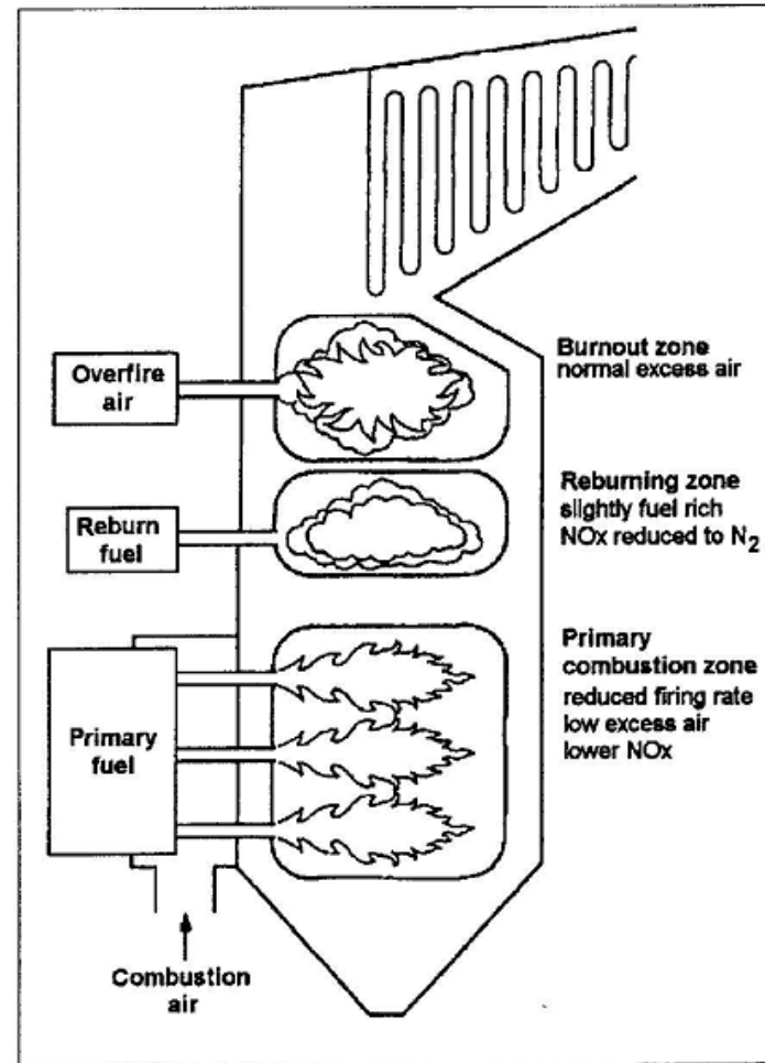
Fig.A4.13: Schema di "reburning".
