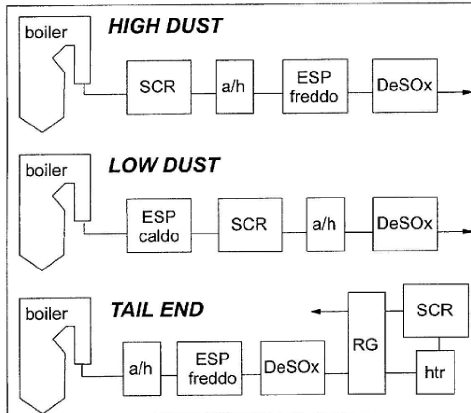
Fig.A4.15: Possibili configurazioni di inserimento di un SCR a valle di un generatore di vapore (boiler). Legenda: a/h: riscaldatore aria comburente; ESP: precipitatore elettrostatico; DeSOx: desolfuratore; RG: scambiatore rigenerativo; htr: post-riscaldatore con combustione di gas naturale.
