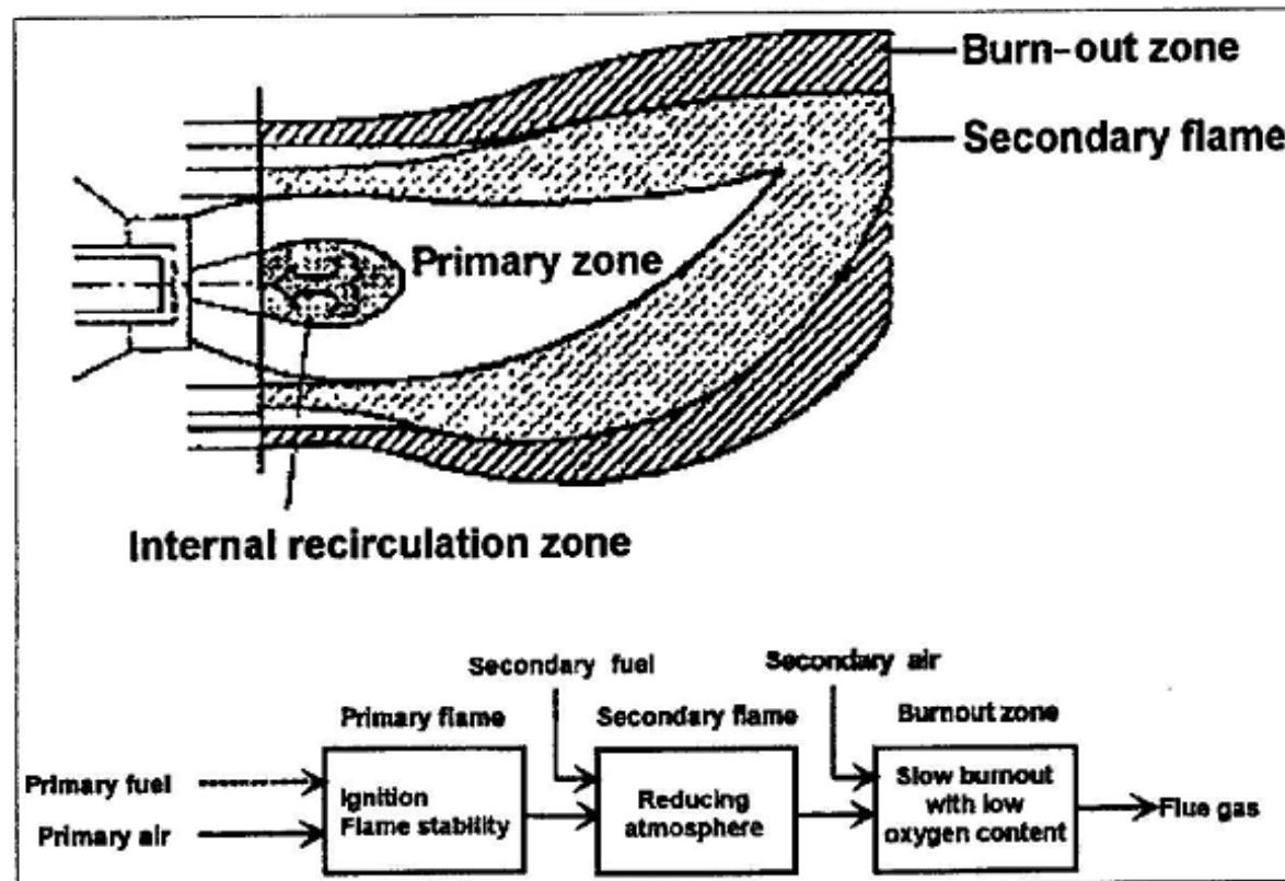
Fig.A4.14: Schema concettuale di bruciatore a bassa emissione di NOx.
