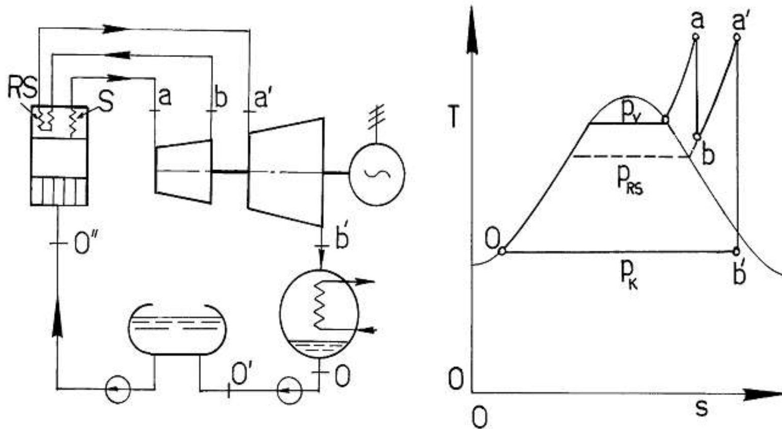
Ciclo a vapore risurriscaldato con condensazione
