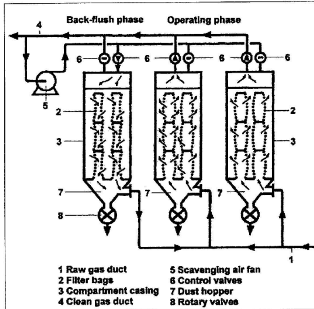
Fig.A4.17: Principio di funzionamento di 'fabric filters'.
