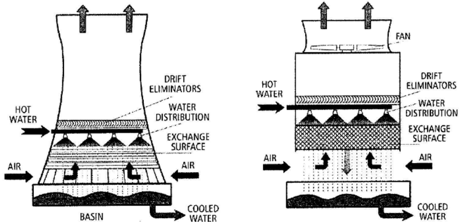
Fig.A4.12: Schemi di torri evaporative. A sinistra una torre a circolazione naturale dell'aria, usata per grandi centrali, a destra una torre a circolazione forzata (induced draft), più diffusa per applicazioni di minore potenza (fonte: Hamon).
