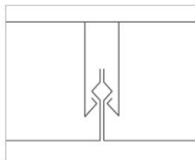
Orditura nascosta
