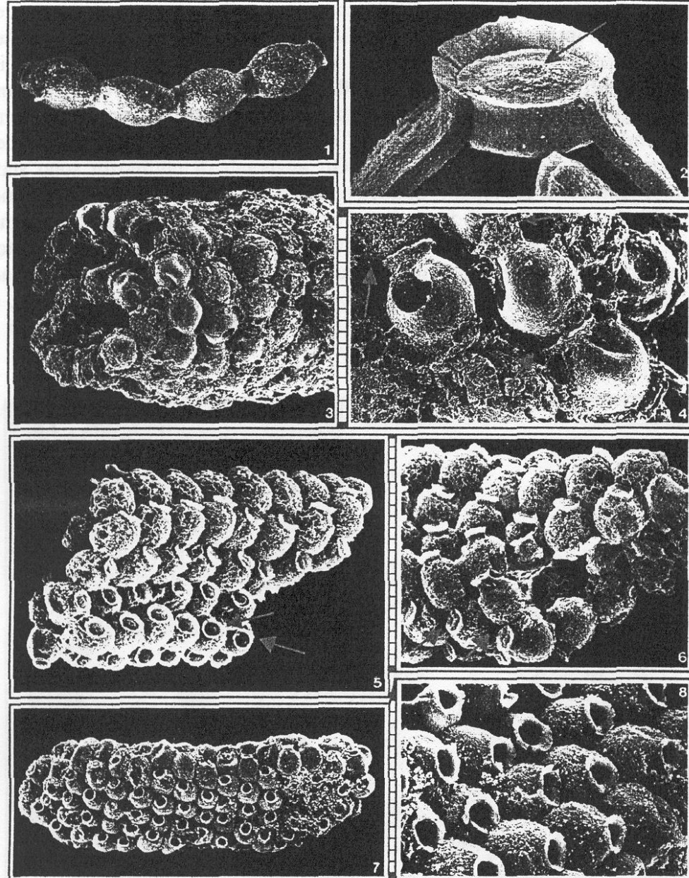
Desmochitina nodosa
