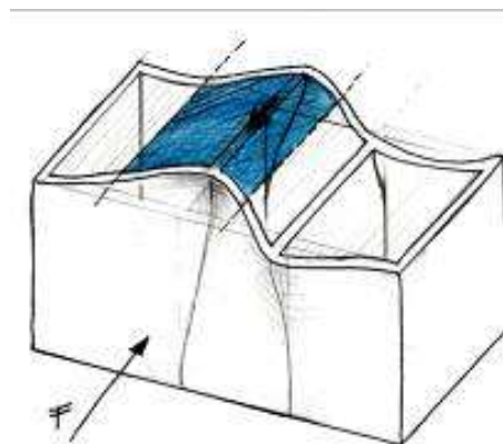
Solaio deformabile
