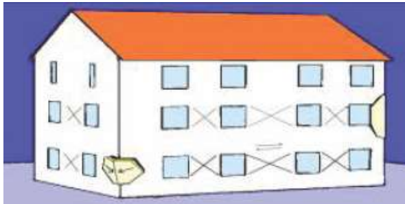
Budva, 1979 - Rottura a taglio dei maschi del piano terra
