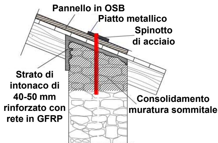
Muratura a singolo paramento
