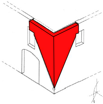
Ribaltamento cantonale
