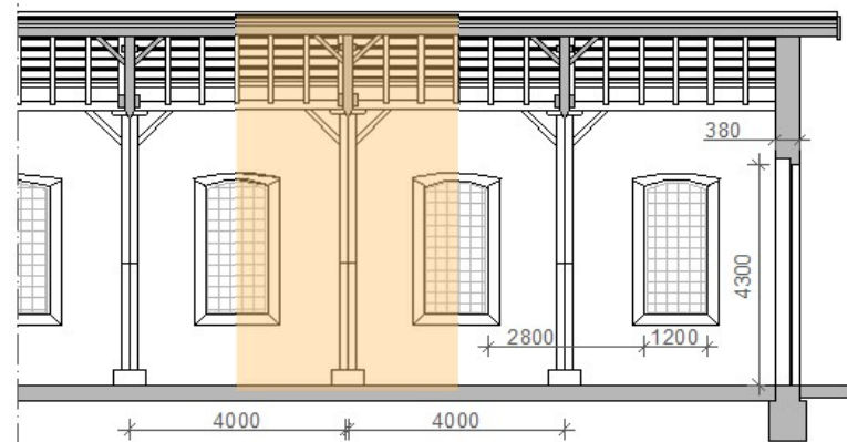
Sezione longitudinale
