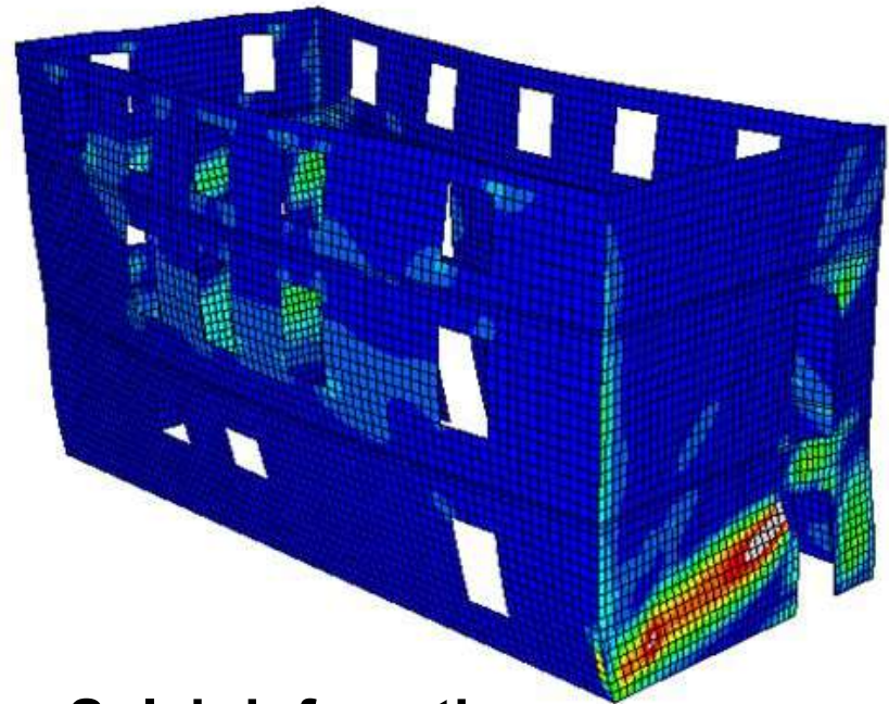
Solai rinforzati
