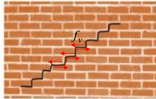
Muratura regolare fessurazione «a scaletta»
