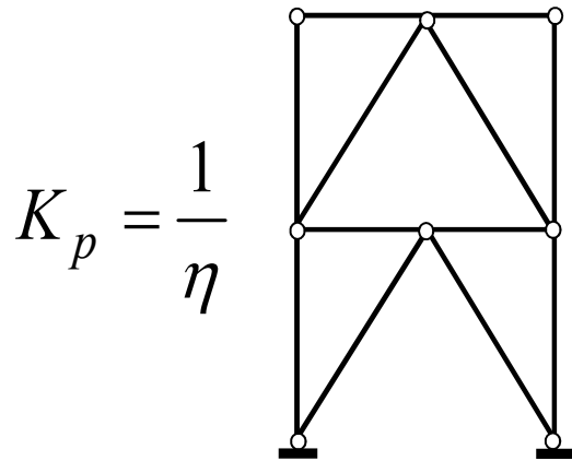
Controvento reticolare in acciaio
