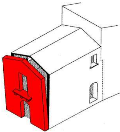
Ribaltamento parete
