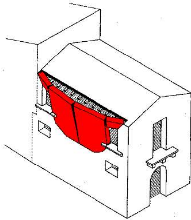
Flessione orizzontale fuori piano
