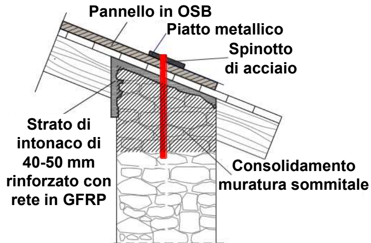
Muratura a singolo paramento
