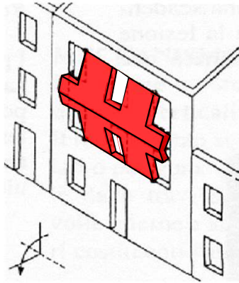
Flessione verticale fuori piano
