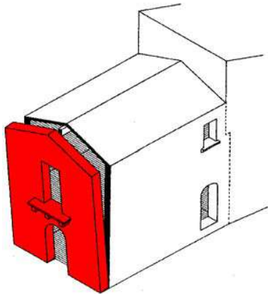
Ribaltamento parete
