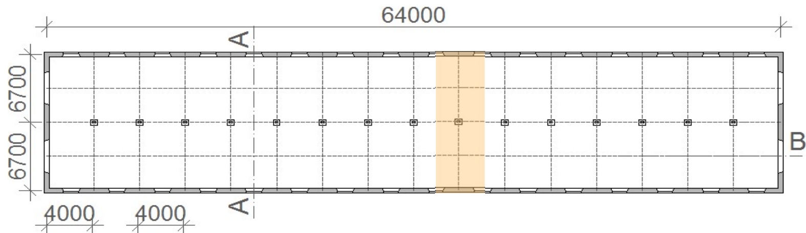
Pianta
