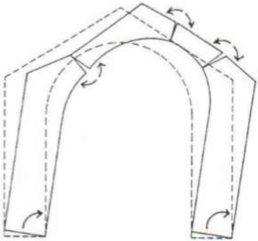
Meccanismo di rottura arco
