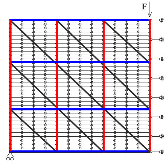
Solaio con nastri in CFRP
