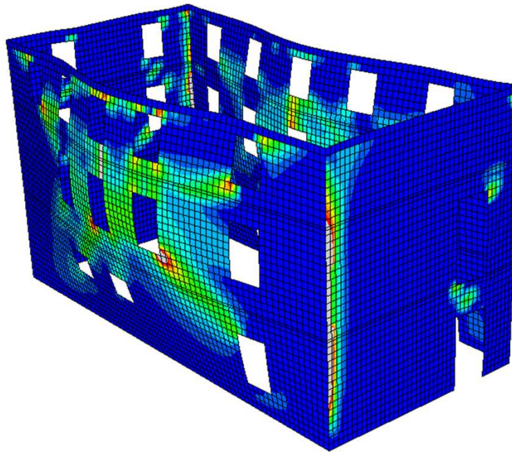
Solai originali
