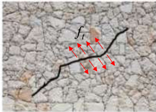
Muratura irregolare fessurazione diagonale
