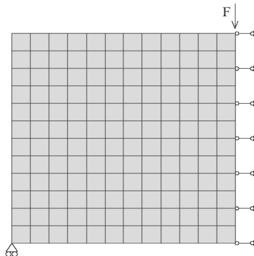
Solaio con soletta in cls
