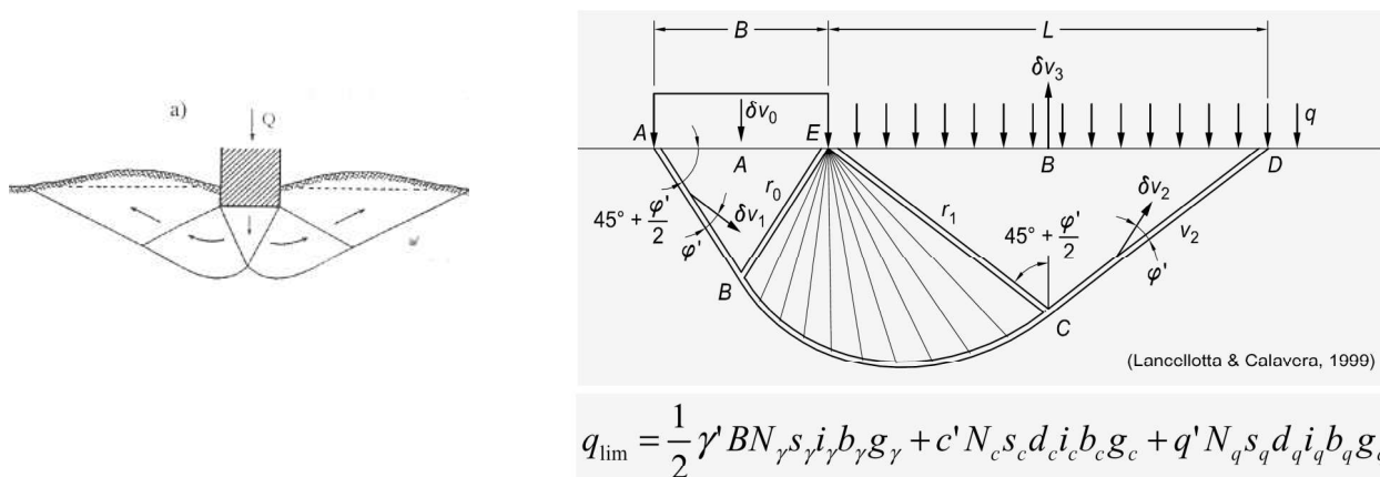
Formula di Brinch-Hansen (statica)
