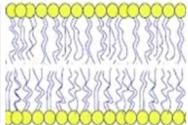
FASE LIQUIDO-CRISTALLINA
