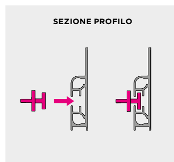
PROFILO CONTINUO in alluminio (già compreso nel prezzo delle basi).
