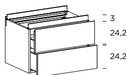
Base 2 cassetti con gola (di serie in alluminio nero) 1° cassetto con interno sagomato
