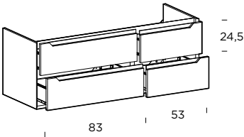
Base portalavabo SX 4 cassetti (1° con int. sagomato)
