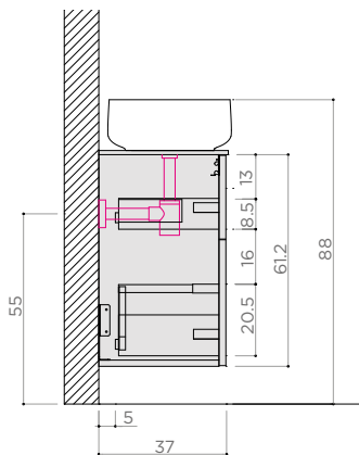
LAVABO "TUTTO FUORI" (con sifone art. 5692) stessa posizione per base con VANO A GIORNO
