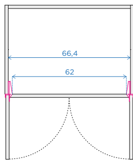
VISTA DALL'ALTO
