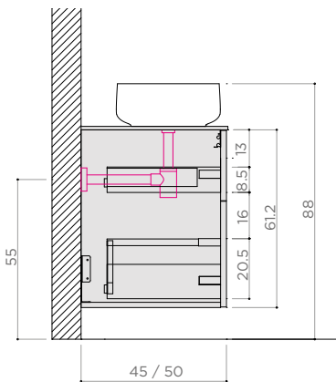
LAVABO "TUTTO FUORI" (con sifone art. 5692) stessa posizione per base con VANO A GIORNO
