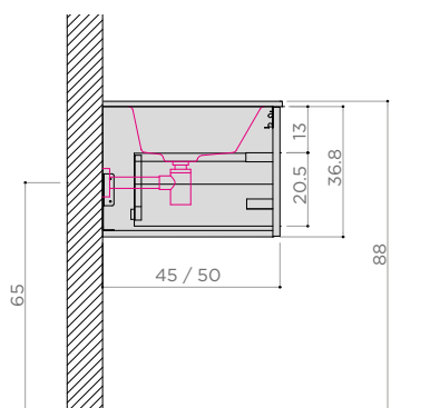
LAVABO INCASSO (con sifone art. 5692)
