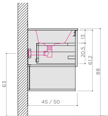
LAVABO INCASSO (con sifone art. 5697) base con VANO A GIORNO
