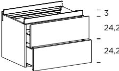
Base portalavabo 2 cassetti con gola (di serie in alluminio nero) 1° cassetto con interno sagomato
