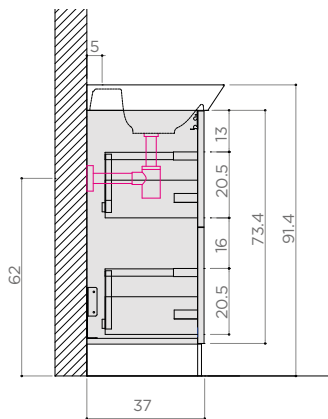
LAVABO CONSOLLE TODAY (con sifone art. 5692)
