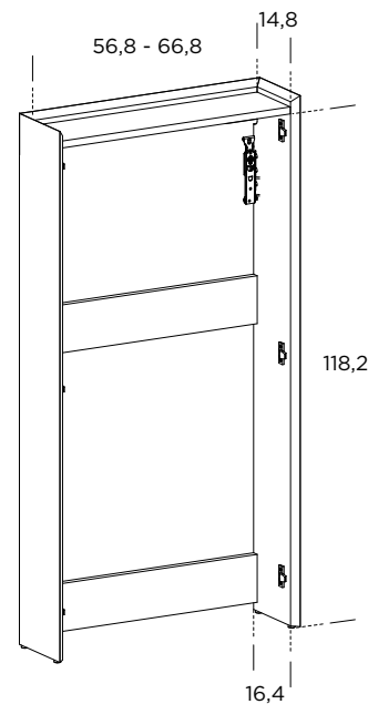
MISURE INTERNE BASE ISPEZIONABILE
