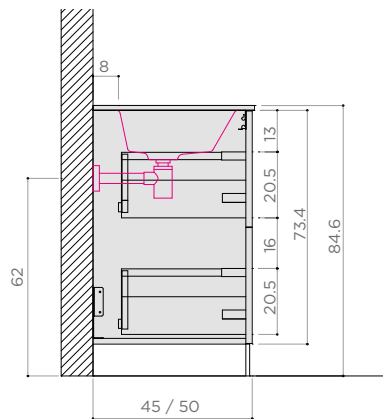
LAVABO INCASSO (con sifone art. 5692)
