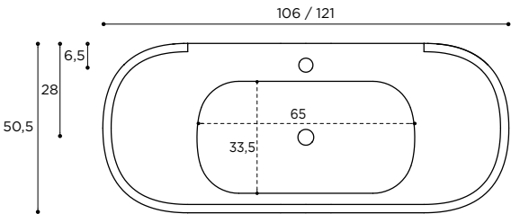
Consolle in Tekno Deimos / Tekno colore sp. 2 cm Vasca interna L 65 x P 33,5 x H 11 cm Finitura in tinta nella parte inferiore Di serie con foro rubinetetto, a richiesta senza (installare con piletta art. 5698/99/96)
