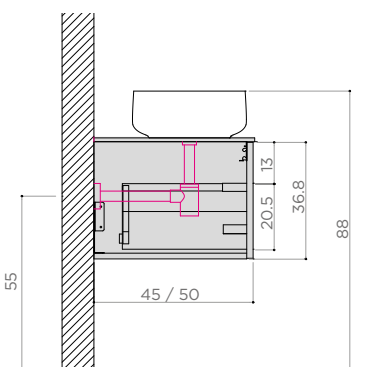
LAVABO "TUTTO FUORI" (con sifone art. 5692)
