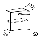
Base terminale 1 anta dx-sx
