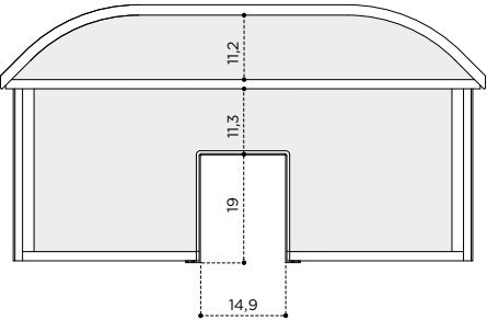
Sagomatura per BASI MOBY
