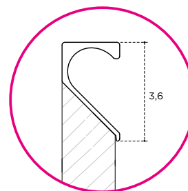
SEZIONE MANIGLIA
