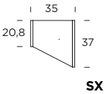
Base terminale a giorno dx-sx (ripiano legno fisso)
