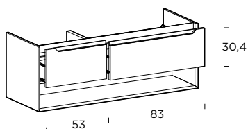
Base portalavabo DX 2 cassetti (int. sagomato) 1 vano a giorno
