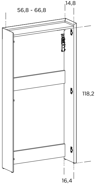
MISURE INTERNE BASE ISPEZIONABILE
