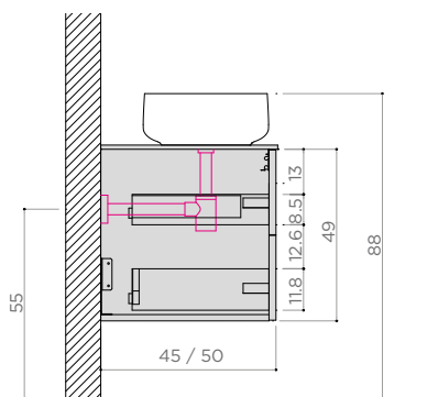
LAVABO "TUTTO FUORI" (con sifone art. 5692)
