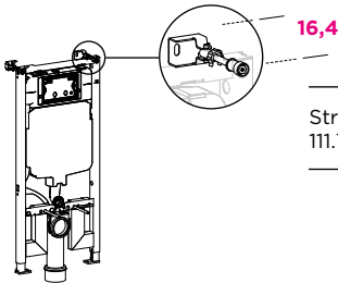
Base per WC
