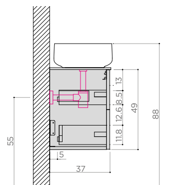
LAVABO "TUTTO FUORI" (con sifone art. 5692)
