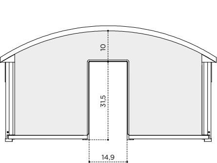
Sagomatura per BASI FUSION
