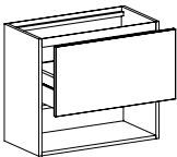
Base portalavabo 1 cassetto H 36,8 cm con vano a giorno
