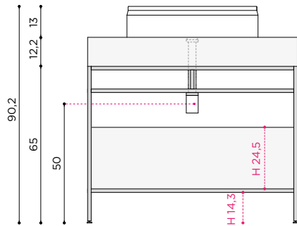
SCATOLATO H 12,2 cm + LAVABO "TUTTO FUORI"
