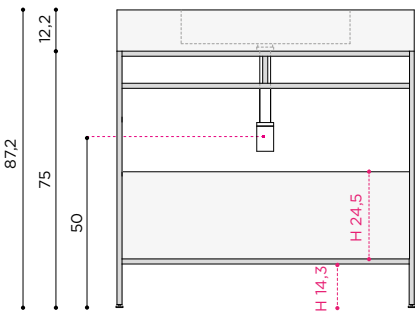
SCATOLATO H 12,2 cm + LAVABO INTEGRATO
