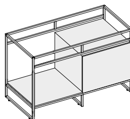
PIANO TOP sp. 1,2 cm + BASE H 36,8 cm (L 50 o 70 cm + top)
