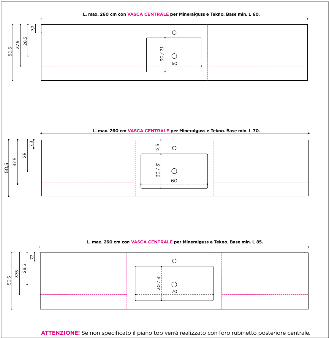
VERSIONE TEKNO COLORE (colori della mazzetta Arbi esclusi metal) Sp. 8 cm
