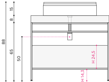
SCATOLATO H 8 cm + LAVABO "TUTTO FUORI"
