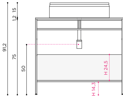
TOP sp. 1,2 cm + LAVABO "TUTTO FUORI"
