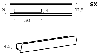
Mensole Slide in alluminio con foro portasalviette L 30 x P 4 cm dx-sx
