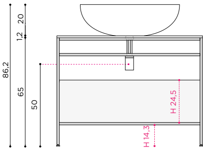
TOP sp. 1,2 cm + LAVABO "TUTTO FUORI"
