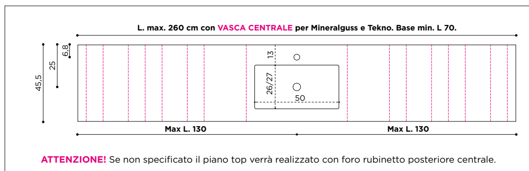
VERSIONE TEKNO COLORE (colori della mazzetta Arbi esclusi metal) Sp. 8 cm
