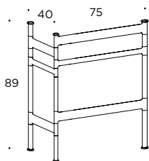
Portasalviette in legno massello
