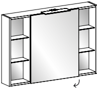
Specchiera Side con 1 anta specchio dx-sx con specchio interno Faretto Flash (art. V818) 2 vani a giorno con 2 spot led (1 W)
