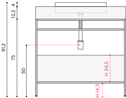
SCATOLATO H 12,2 cm + LAVABO "SOPRAPIANO"
