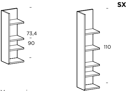
Vano a giorno con 4-5 ripiani sospeso. Dx-sx
