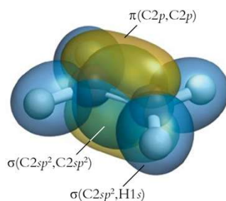
Figura 2F.12 Vista dello schema di legame nell'etene (etilene), che mette in evidenza l'intelaiatura di legami \sigma e il singolo legame \pi formato dalla sovrapposizione laterale di due orbitali \text{C}2p non ibridi. Il doppio legame resiste alla torsione, perché questa diminuirebbe la sovrapposizione tra i due orbitali \text{C}2p , indebolendo il legame \pi . La struttura del legame è sovrapposta a un modello ad aste e sfere.
