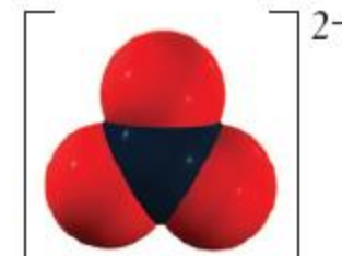
Ione carbonato, \text{CO}_3^{2-}
