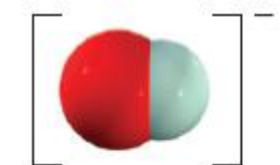
Ione idrossido, \text{OH}^-
