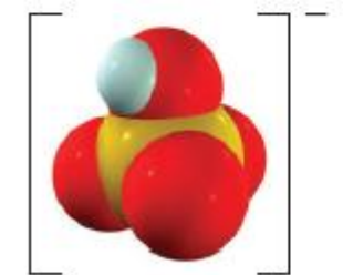
Ione bisolfato, \text{HSO}_4^-
