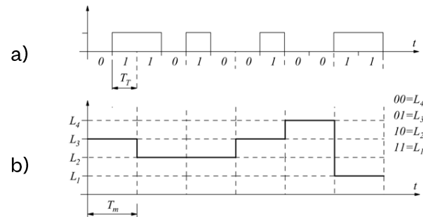
a) Segnale digitale-binario; b) Segnale multi-livello 2^n=4
