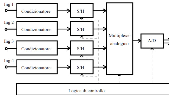
SAD multicanale a campionamento simultaneo con singolo convertitore.
