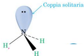
Ammoniaca
