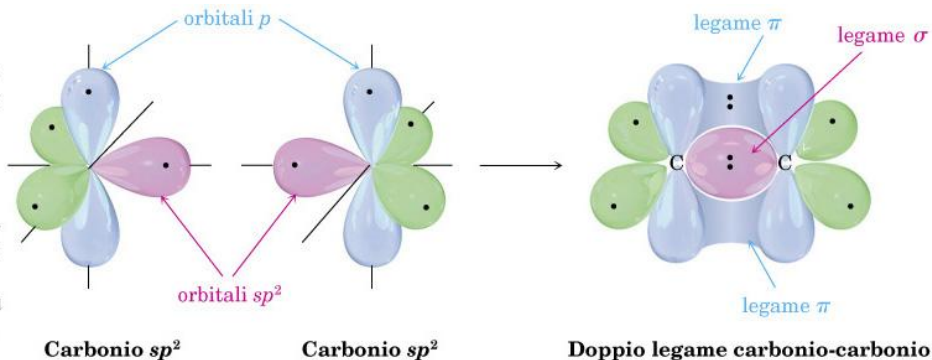
FIGURA 1.14 Sovrapposizione orbitalica di due atomi di carbonio ibridizzati sp^2 a formare un doppio legame carbonio-carbonio. Una parte del doppio legame deriva dalla sovrapposizione \sigma (testa-testa) degli orbitali sp^2 (rosso), e l'altra parte deriva dalla sovrapposizione \pi (laterale) degli orbitali p non ibridizzati (blu). Il legame \pi ha regioni di densità elettronica su ciascun lato di una linea tracciata tra i nuclei.
