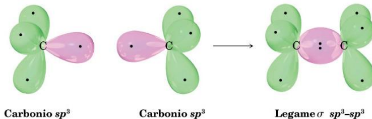
FIGURA 1.12 Struttura dell'etano. Il legame carbonio-carbonio viene formato per sovrapposizione \sigma di due orbitali ibridi sp^3 . (Per chiarezza, i lobi più piccoli degli orbitali ibridi sp^3 non vengono mostrati).
