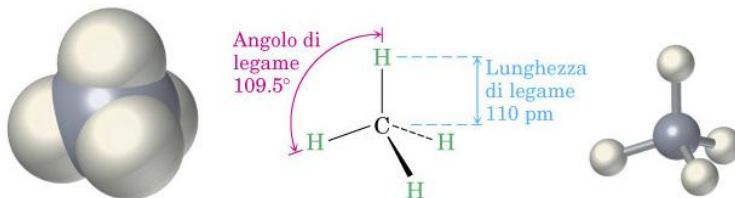
FIGURA 1.11 Struttura del metano che mostra gli angoli di legame di 109.5^\circ .
