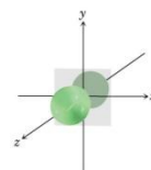
Orbitale 2p_z
