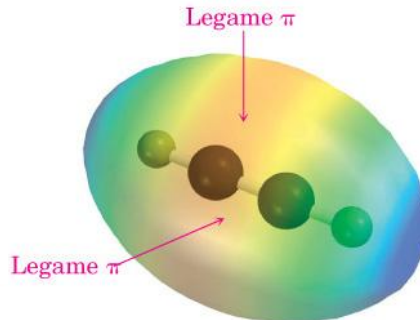
FIGURA 8.1 Struttura dell'acetilene.
