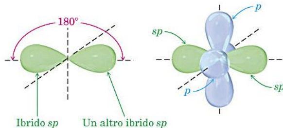
FIGURA 1.16 Un atomo di carbonio ibridizzato sp . I due orbitali ibridi sp (verde) sono orientati a 180^\circ l'uno dall'altro, e sono perpendicolari ai due orbitali p rimanenti (blu).
