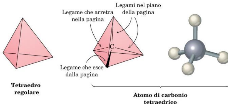
FIGURA 1.6 L'atomo di carbonio tetraedrico secondo van't Hoff. Le linee continue giacciono nel piano della pagina, la linea a cuneo pieno esce dal piano della pagina, e la linea tratteggiata va all'interno della pagina.
