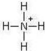
Ione ammonio
