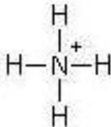
Ione ammonio
