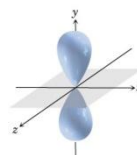
Orbitale 2p_y
