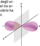
Orbitale 2p_x
