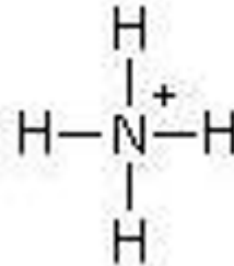
Ione ammonio
