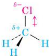
Clorometano
