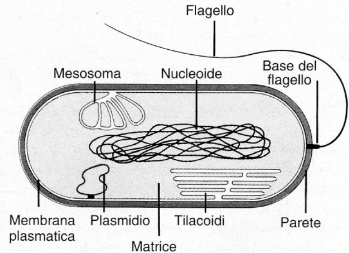
Figura 1.5 Schema di una cellula batterica.
