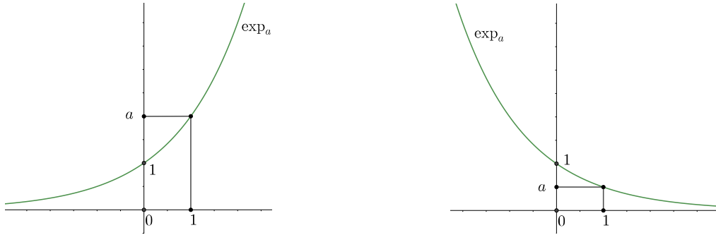
Figure 1: La funzione \exp_a con a > 1 e a < 1 , rispettivamente.
