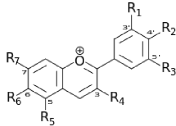
Il catione FLAVILIO , struttura base degli antociani.
