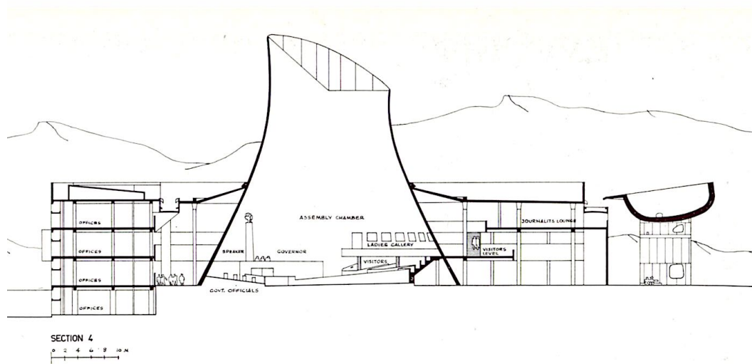
salle d'Assemblée Section through the Assembly Hall Schnitt durch das Parlamentsgebäude
