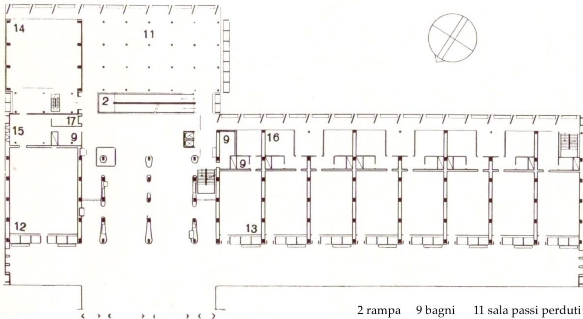
Niveau 2: niveau principal cours et Pas-perdus
