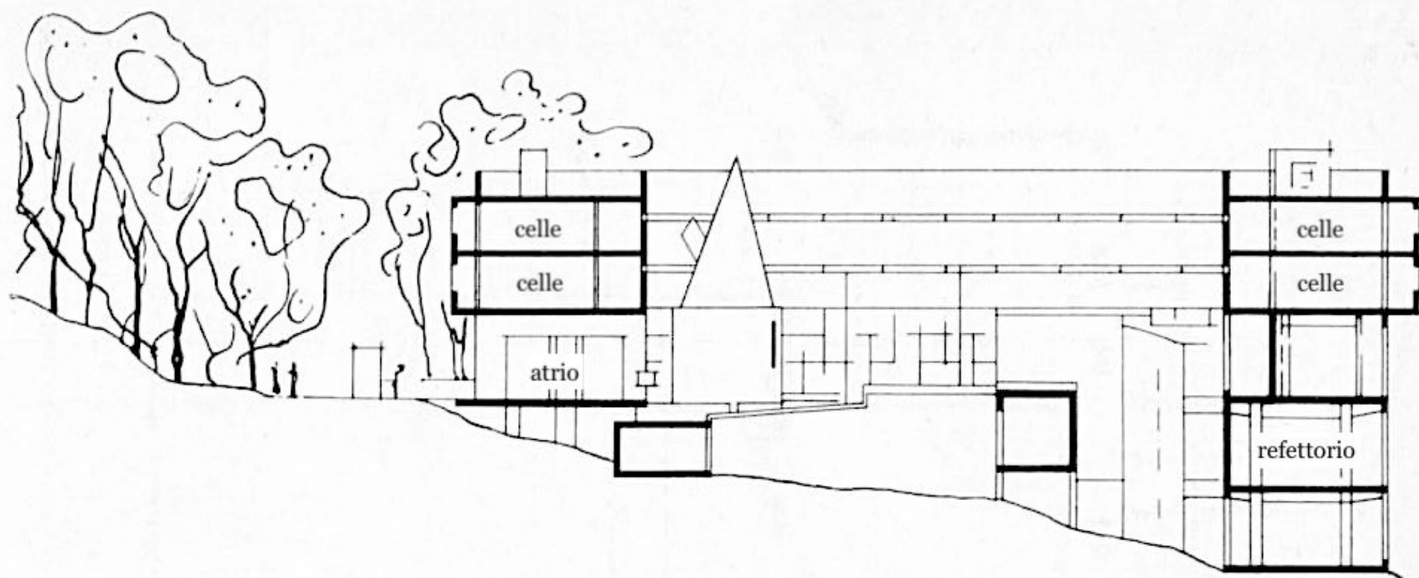
Coupe sur le nouveau couvent
