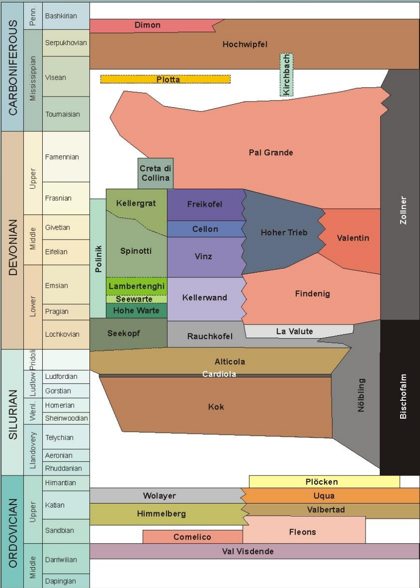
Le unità litostratigrafiche (tutte formazioni) della sequenza Pre-Varisica delle Alpi Carniche
