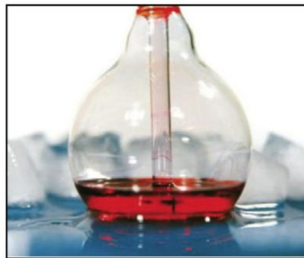
ghiaccio fondente
