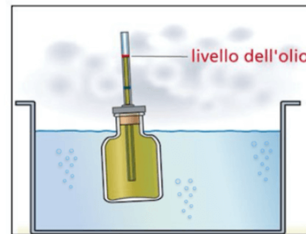
Acqua bollente
