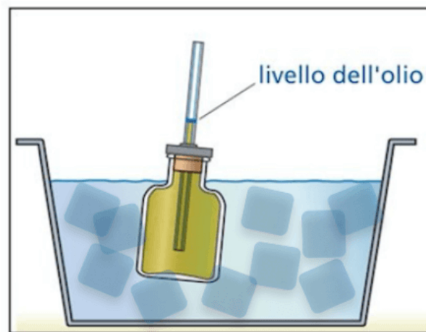
Ghiaccio fondente
