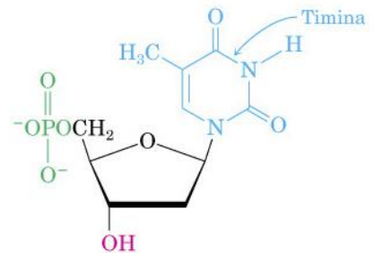
2'-Deossitimidina 5'-fosfato
