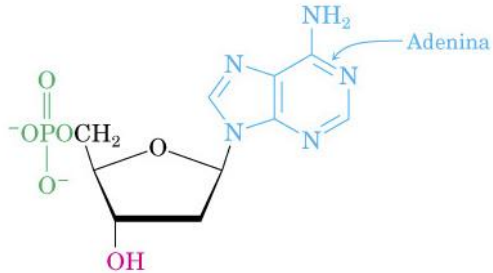
2'-Deossiadenosina 5'-fosfato
