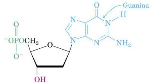
2'-Deossiguanosina 5'-fosfato
