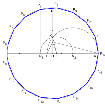
L'eptadecagono
