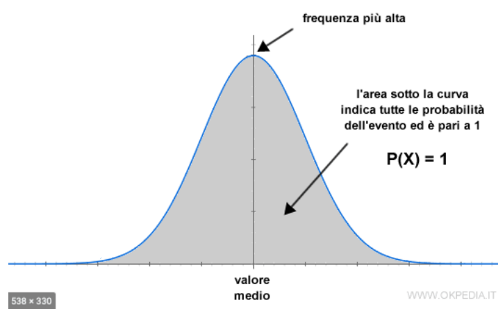
Curva gaussiana
