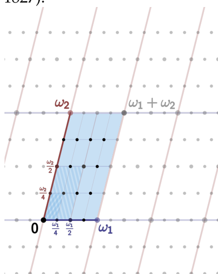
Reticolo fondamentale
