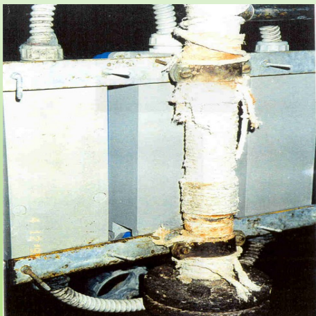
tubo rivestito di cordone di amianto ai fini di isolamento termico
