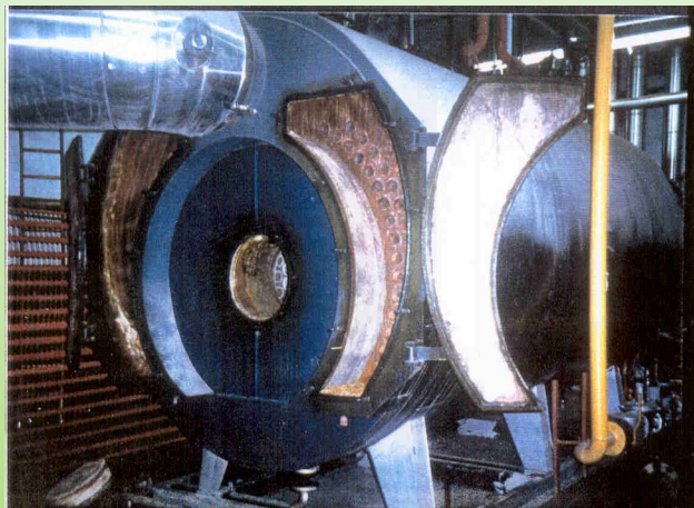
rivestimento di amianto del portellone della caldaia industriale
