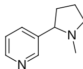
nicotina
