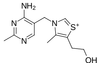
tiamina
