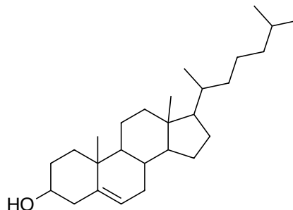
colesterolo
