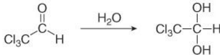
Cloralio idrato
