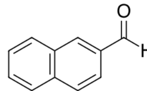
2-naftalenecarbaldeide
