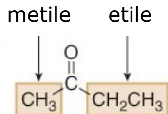
COMUNE etilmetilchetone
