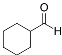
Cicloesancarbaldeide
