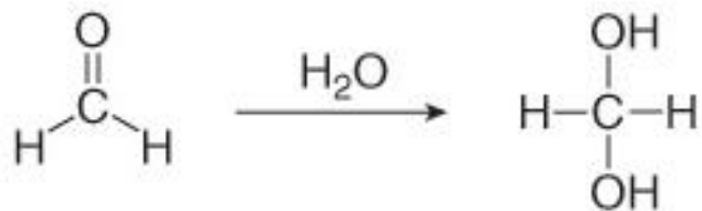
Formaldeide
