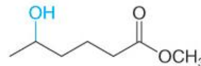
Metil 5-idrossiesanoato
